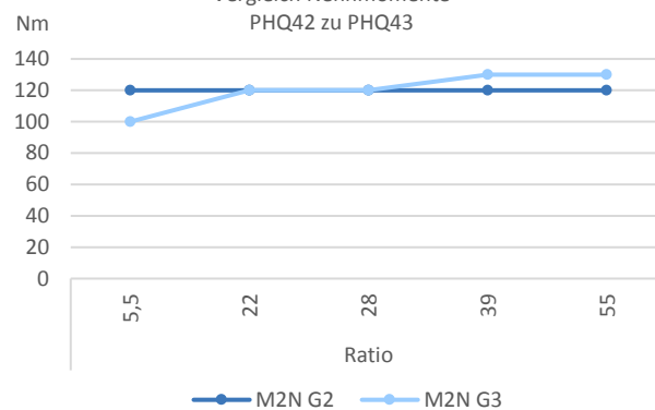
Vergleich Nennmomente PHQ42 zu PHQ43
