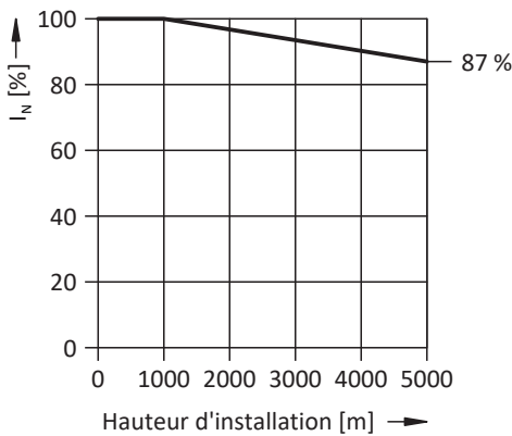
Fig. 21: R duction du courant nominal en fonction de la hauteur d'installation
