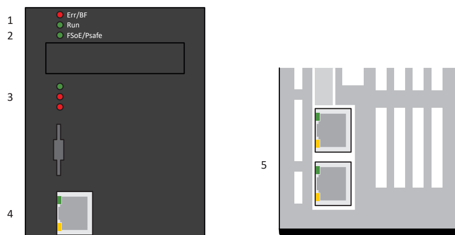
Fig. 86: Positionnement des diodes électroluminescentes de diagnostic sur la face avant et dessus du servo-variateur
