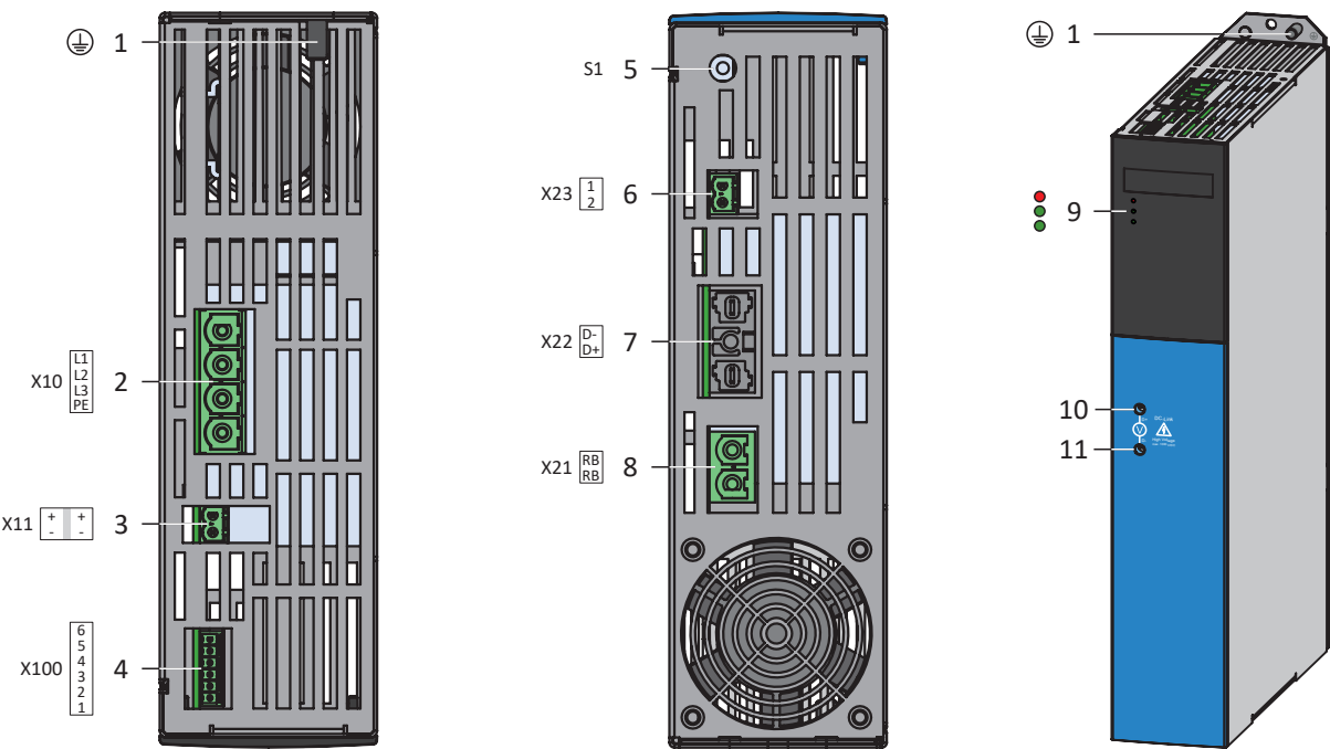
Fig. 46: Schéma de raccordement à l'exemple du PS6A34
