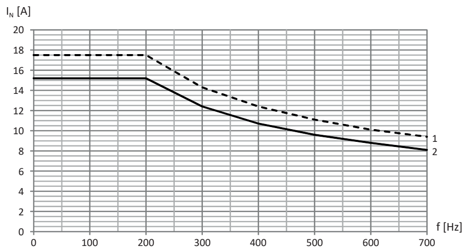
Fig. 24: Réduction du courant nominal en fonction de la cadence, TEP3820-0CS41
