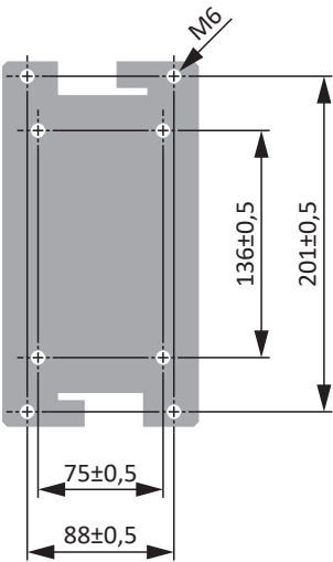
Fig. 41: Plan de perçage self de réseau
