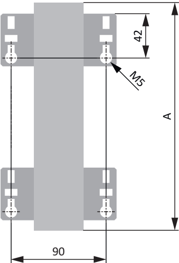
Fig. 38: Plan de perçage KWADQU avec MWS 310L
