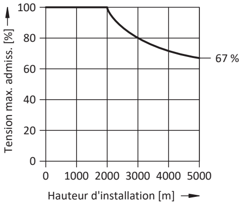
Fig. 22: R duction de la tension en fonction de la hauteur d'installation
