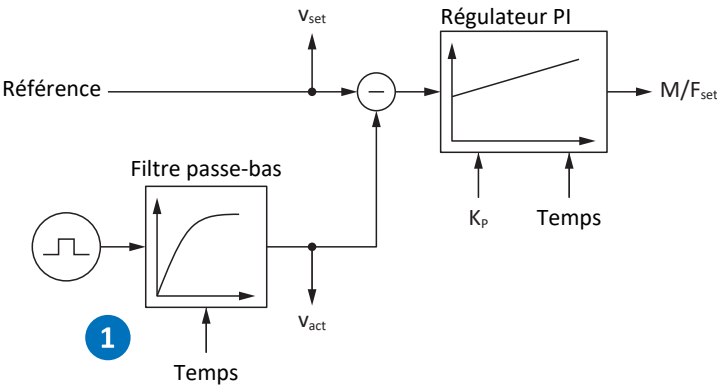
Fig. 60: Régulateur de vitesse – filtre pour la vitesse réelle
