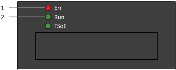
Fig. 88: DEL indiquant l'état EtherCAT
