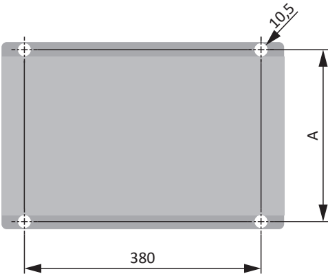
Fig. 40: Plan de perçage FGFKQU
