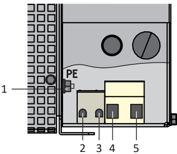
Fig. 53: Schéma de raccordement FGFKQU
