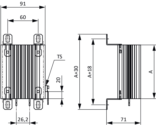
Fig. 13: Croquis coté KWADQU avec MWS306L
