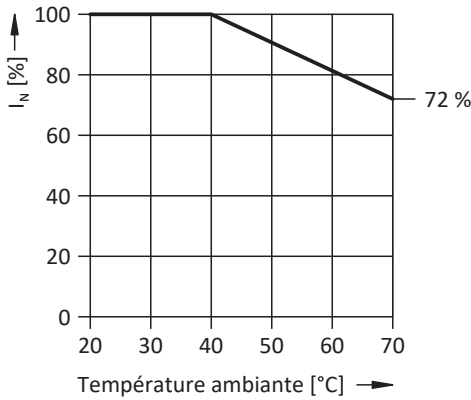
Fig. 20: R duction du courant nominal en fonction de la temp rature ambiante
