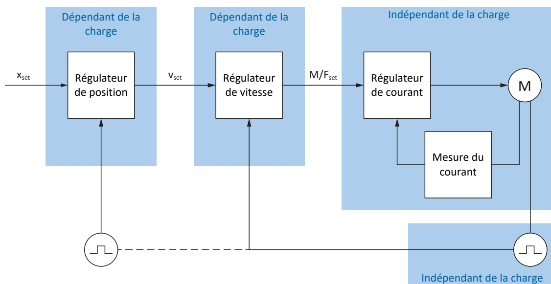
Fig. 58: Structure de la cascade de régulation
