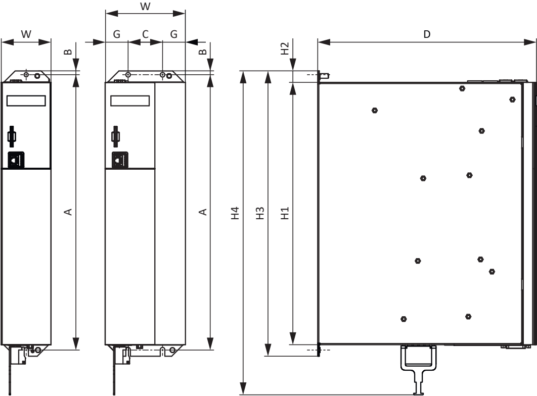
Fig. 10: Croquis coté SI6
