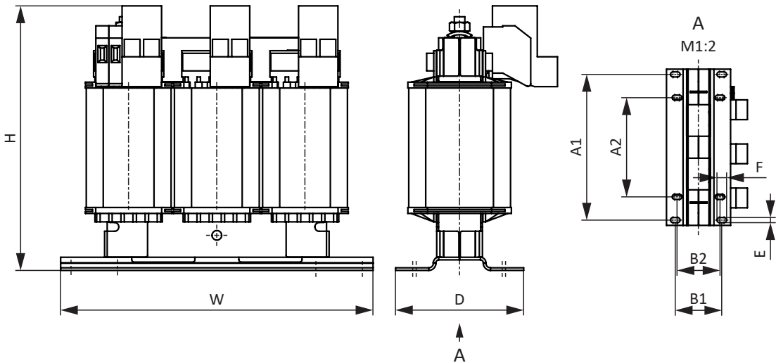
Fig. 5: Esquema de dimensiones TEP
