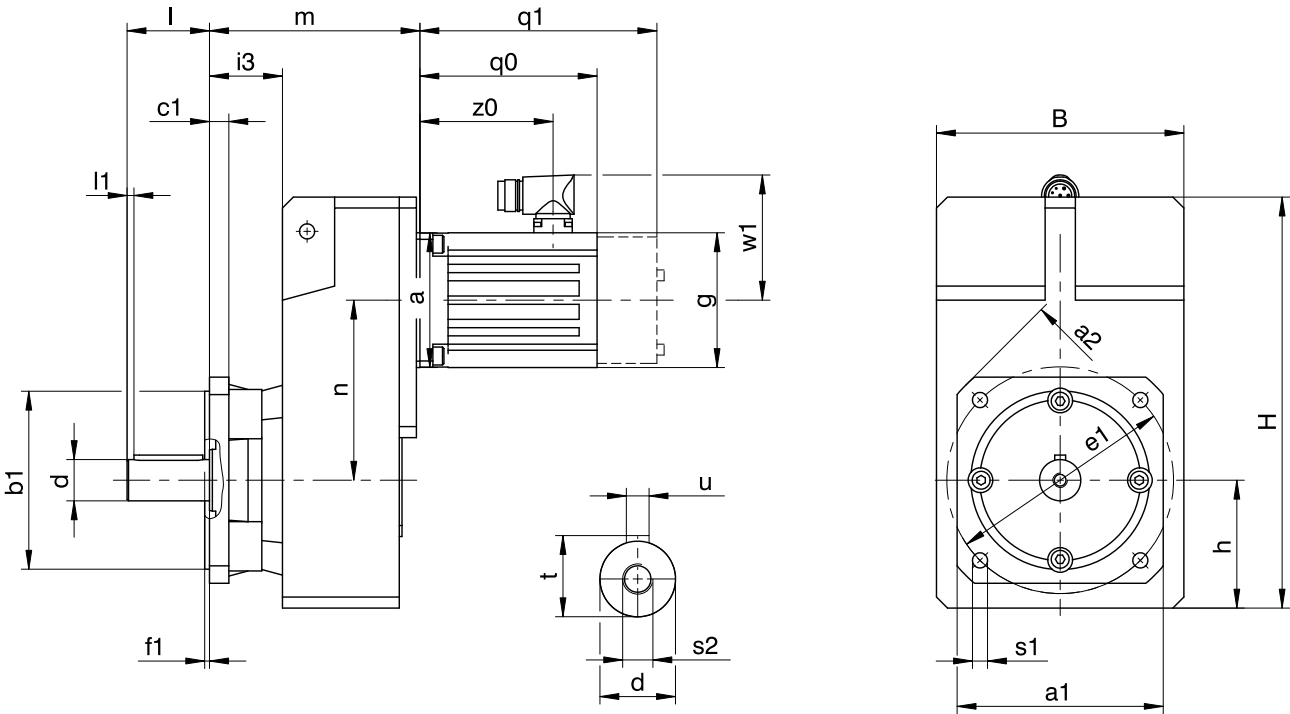
Medidas de los reductores
