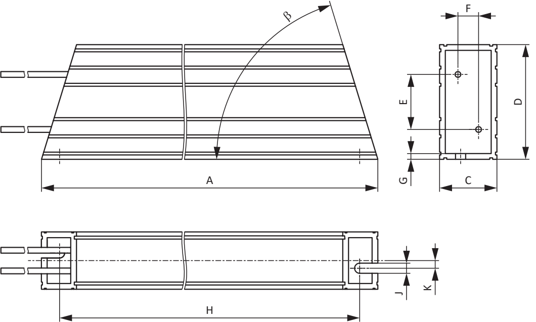
Fig. 5: Esquema de dimensiones GVADU, GBADU
