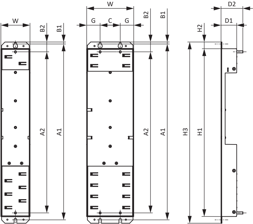
Fig. 5: Esquema de dimensiones DL6B10 hasta DL6B21
