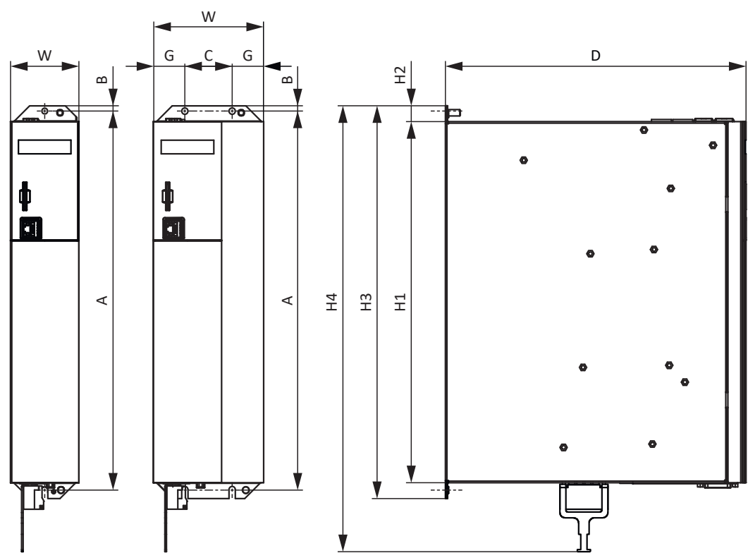
Fig. 4: Esquema de dimensiones SI6
