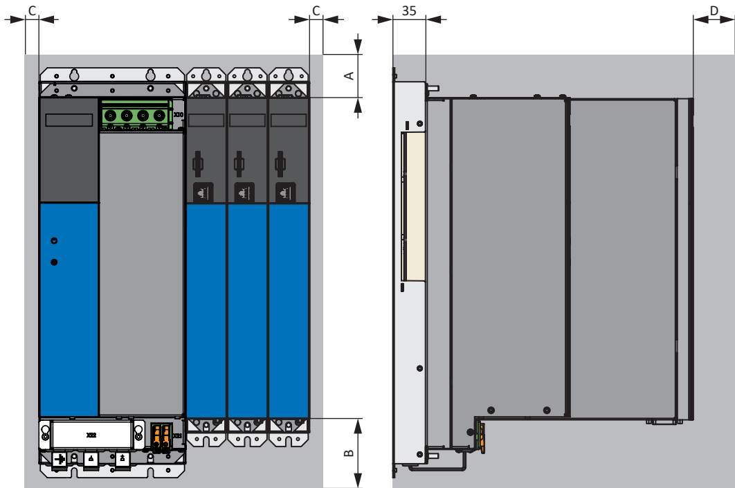
Fig. 8: Espacios libres mínimos para los reguladores de accionamiento en combinación con el módulo de alimentación PS6A44
