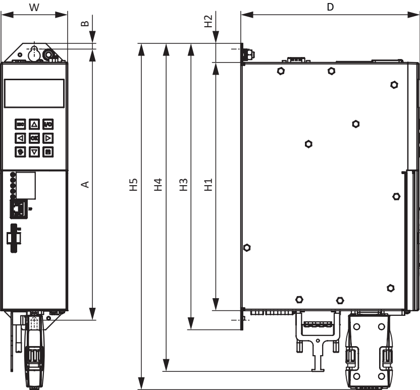
Fig. 1: Esquema de dimensiones SB6
