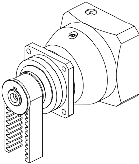
Fig. 3: Asignación recomendada de los rodamientos Z (p. ej., con accionamientos de correa)
