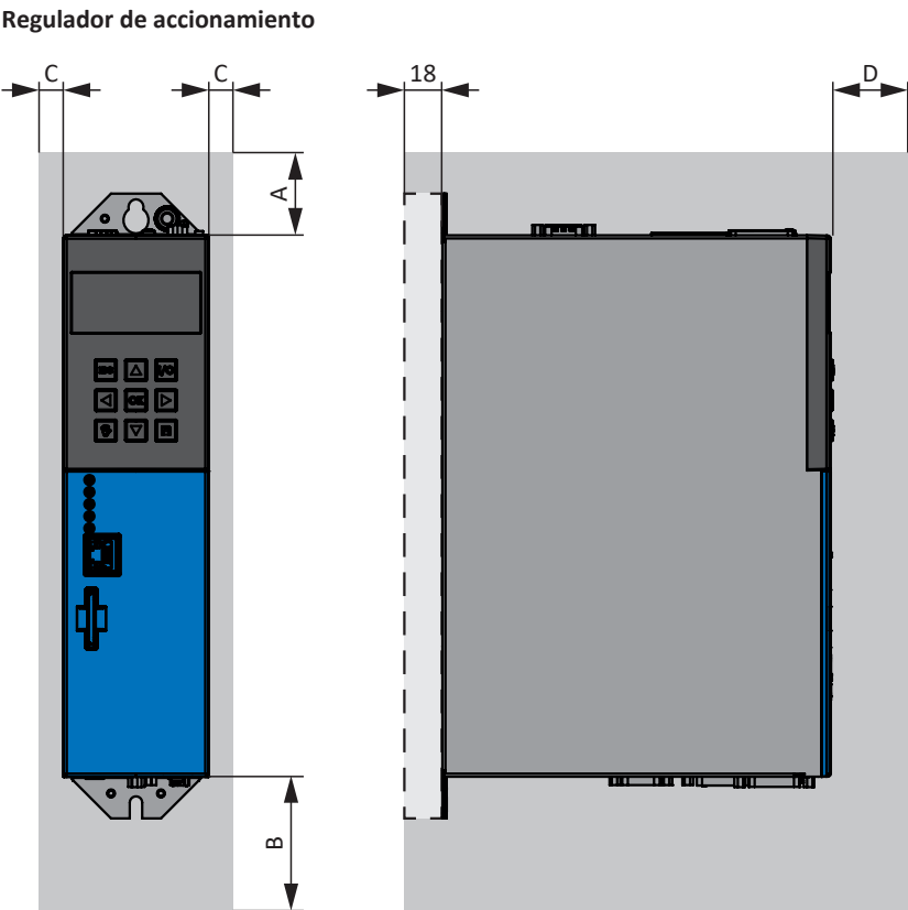
Fig. 2: Espacios libres mínimos
