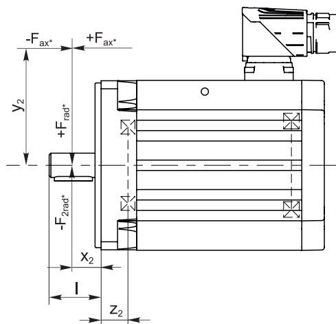
Cargas de los ejes admisibles
