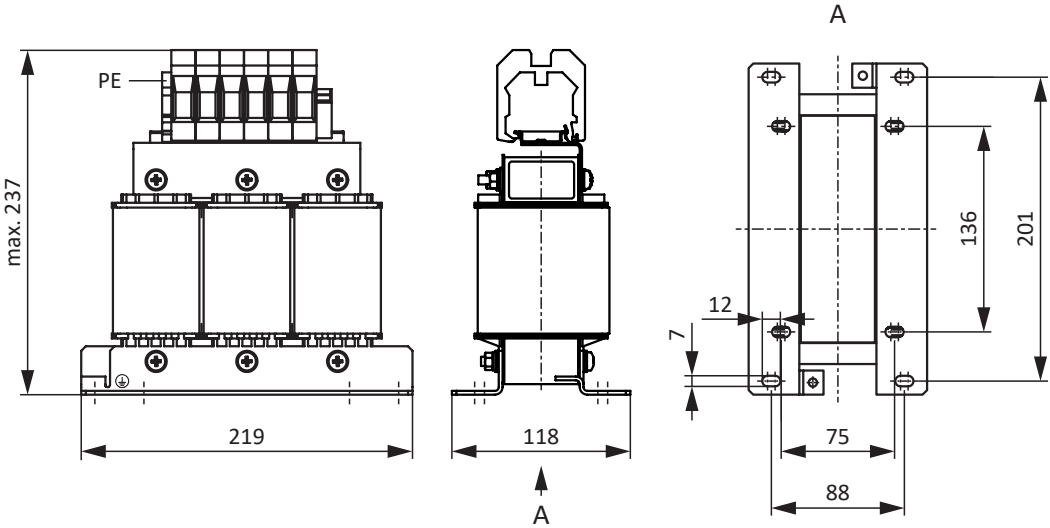
Fig. 13: Esquema de dimensiones estrangulador de red
