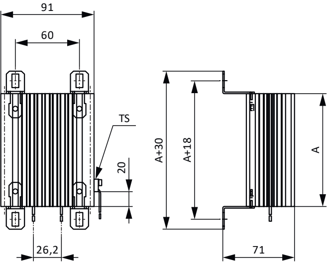
Fig. 9: Esquema de dimensiones KWADQU con MWS306L
