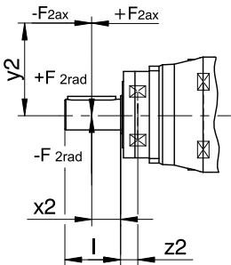
Fig. 4: Puntos de incisión de la fuerza
