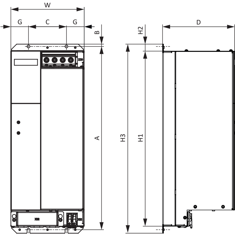
Fig. 2: Esquema de dimensiones PS6A44
