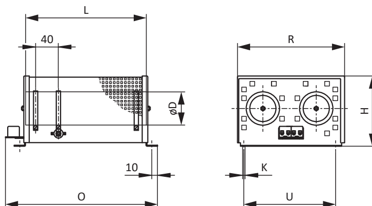
Fig. 11: Esquema de dimensiones FZZMQU
