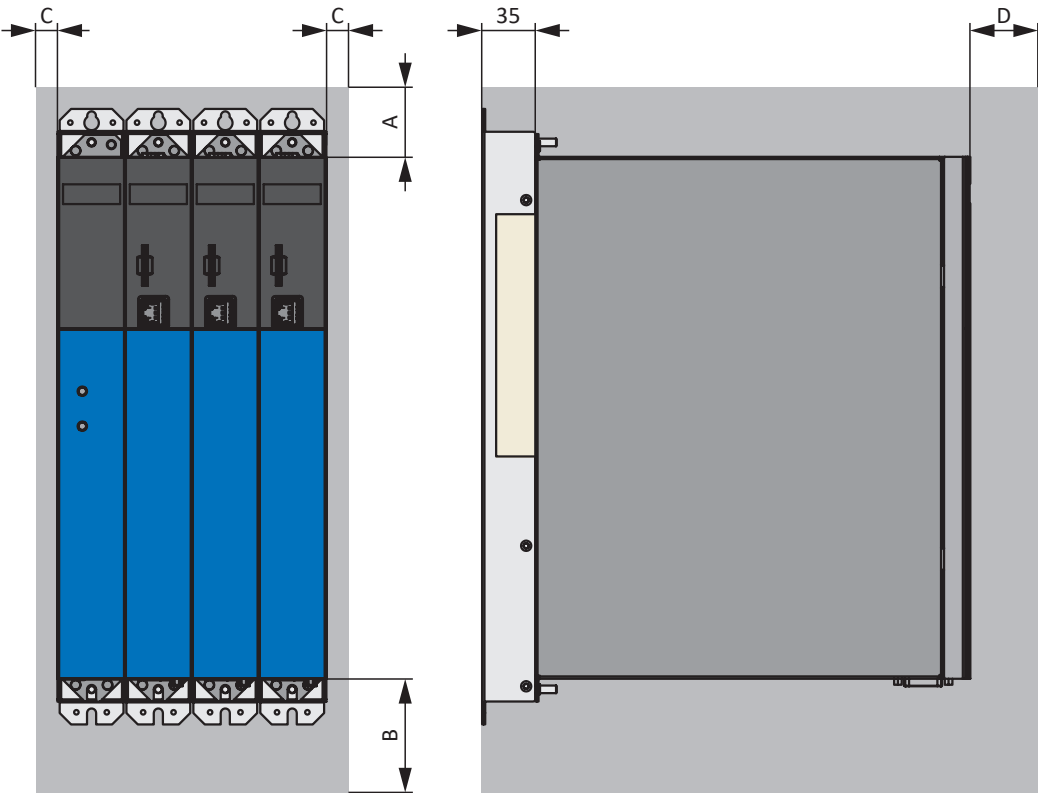
Fig. 7: Espacios libres mínimos para los reguladores de accionamiento en combinación con el módulo de alimentación PS6A24 o PS6A34
