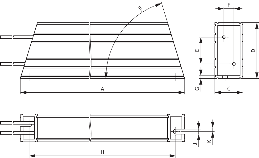
Fig. 4: Esquema de dimensiones GVADU, GBADU
