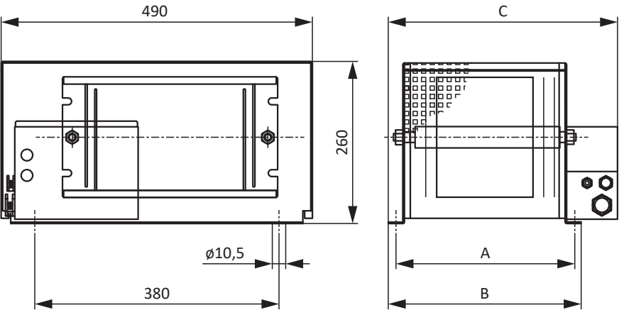
Fig. 12: Esquema de dimensiones FGFKQU
