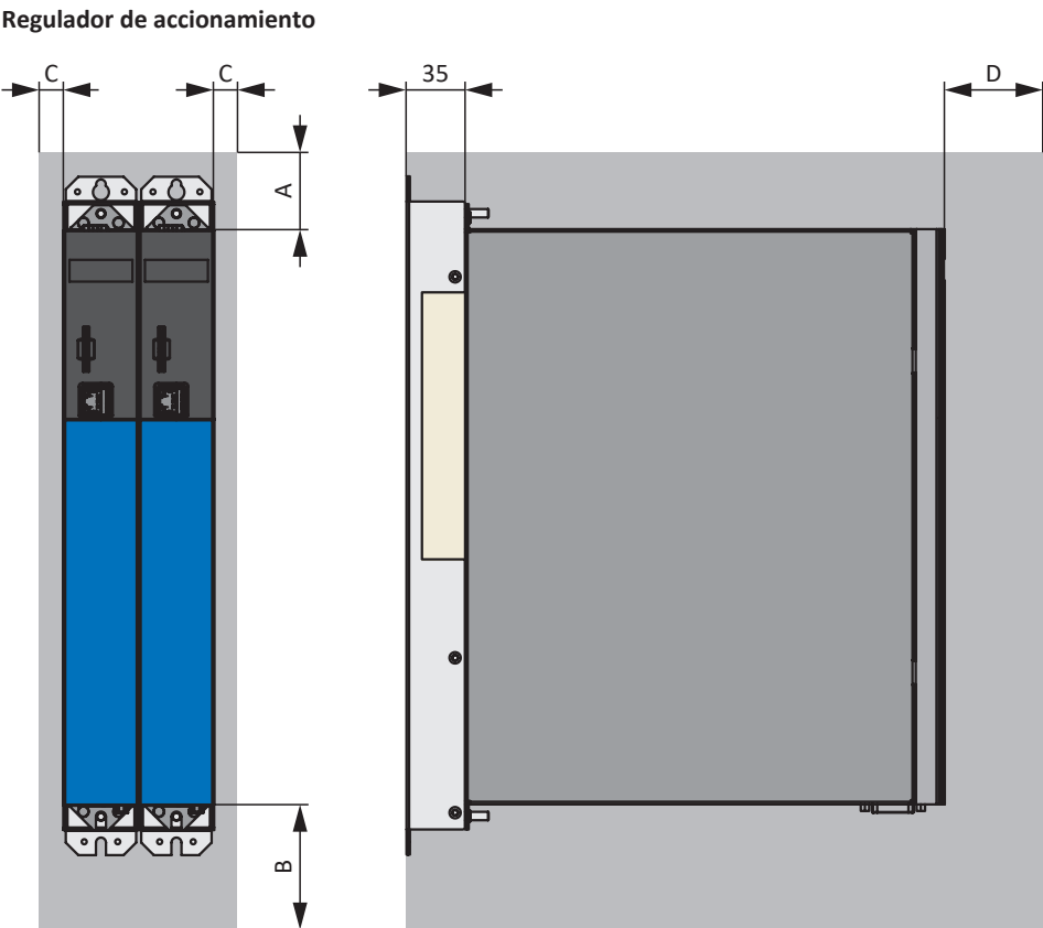
Fig. 3: Espacios libres mínimos
