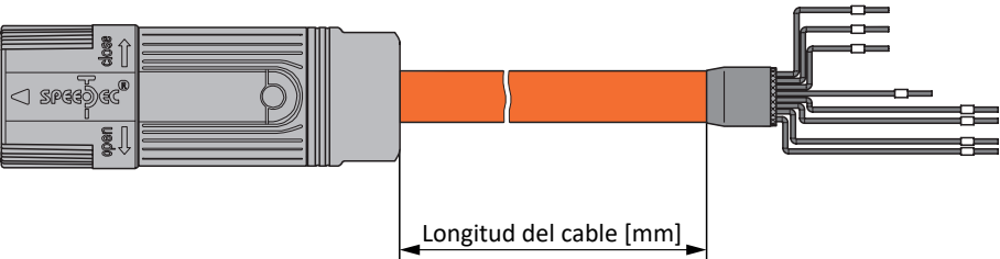
Fig. 1: Definición de longitud para cables de potencia confeccionados
