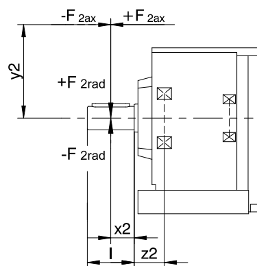
Fig. 1: Puntos de incisión de la fuerza
