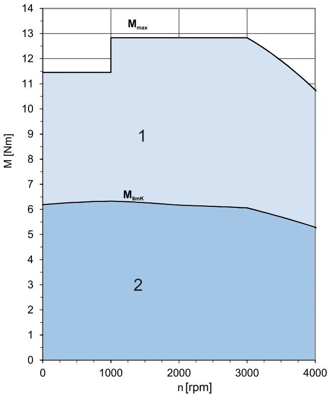
Fig. 1: Explicación de una curva característica del régimen de revoluciones y el par de giro
