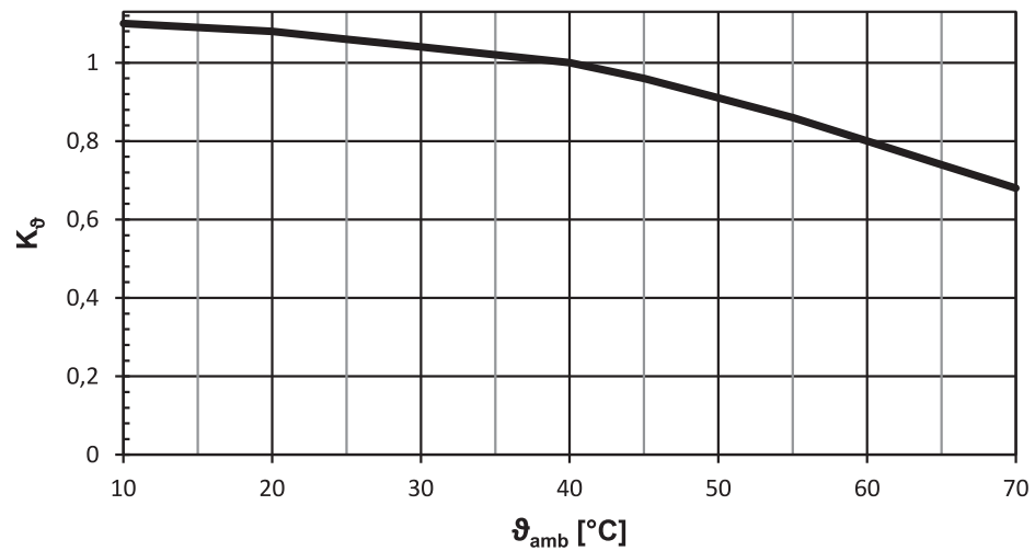
Fig. 4: Reducción de potencia en función de la temperatura ambiente
