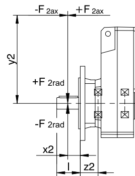
Fig. 1: Puntos de incisión de la fuerza para el eje macizo
