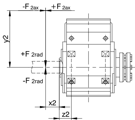
Fig. 2: Puntos de incisión de la fuerza para el eje hueco
