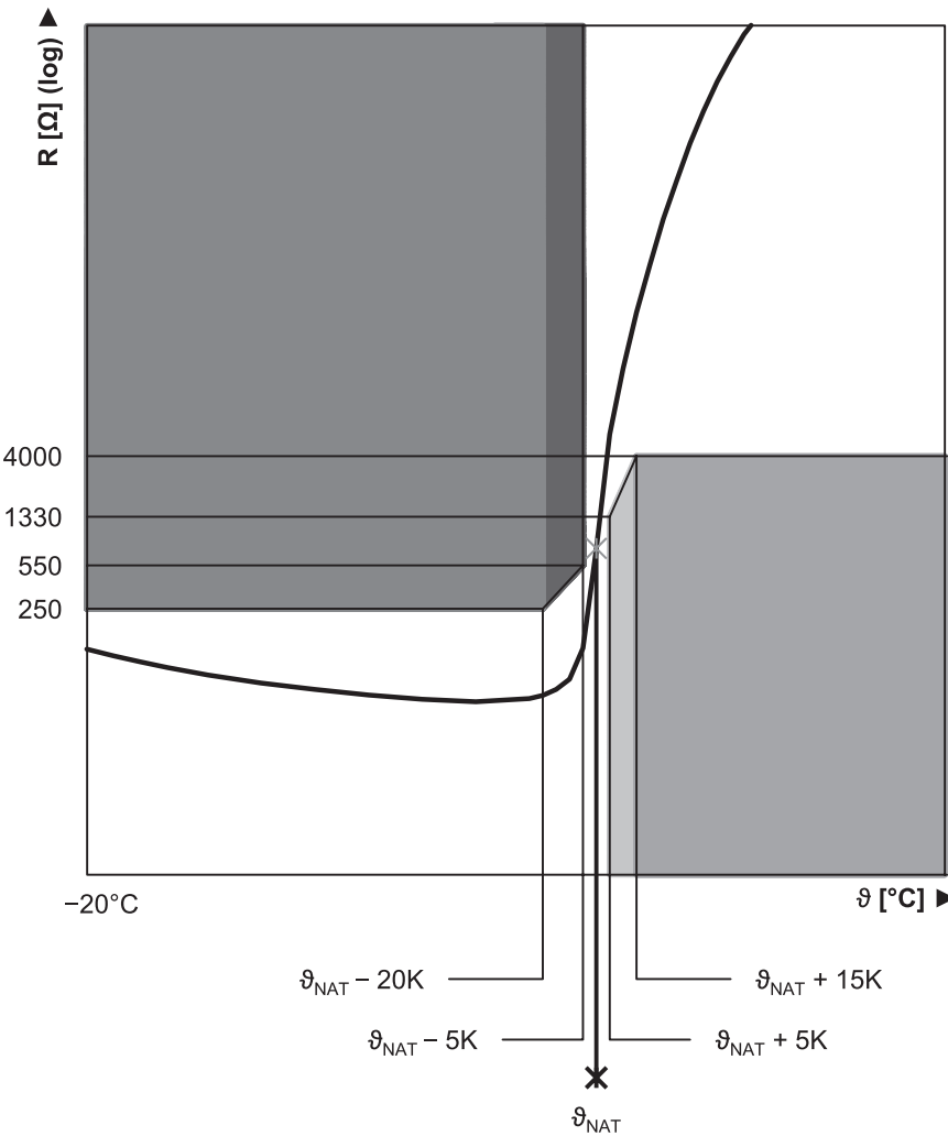
Fig. 2: Curva característica del termistor PTC (un semiconductor frío)
