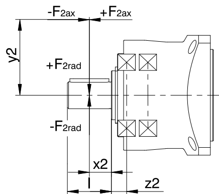
Fig. 1: Puntos de incisión de la fuerza
