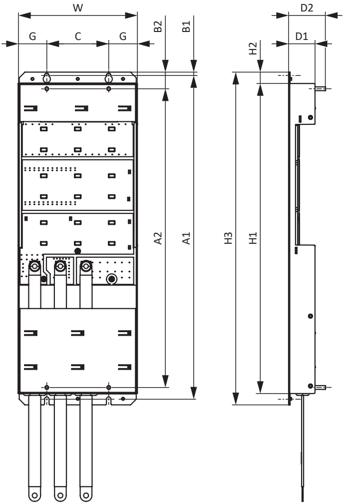
Fig. 6: Esquema de dimensiones DL6B22
