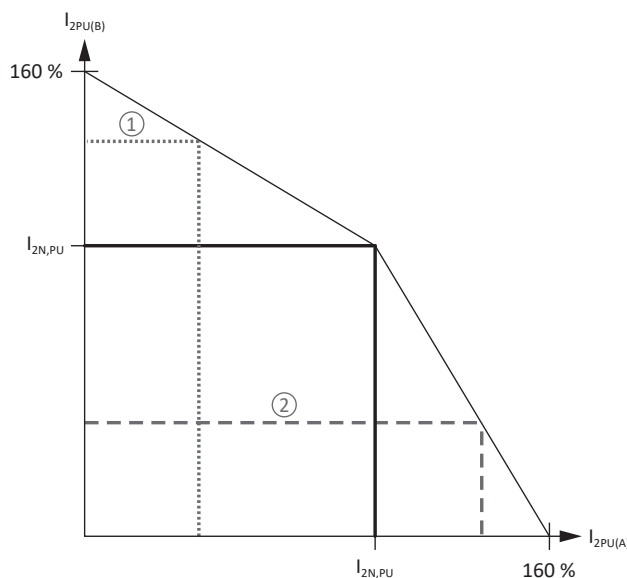
Fig. 1: Carga con terminación simple en reguladores de dos ejes
