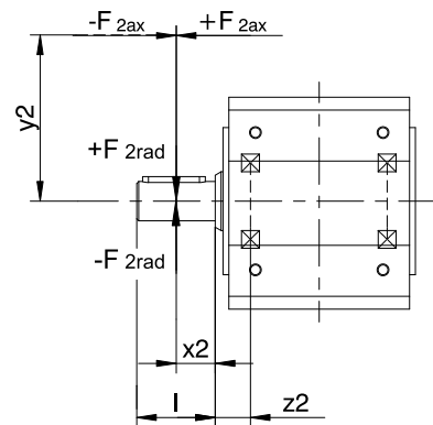
Fig. 1: Puntos de incisión de la fuerza para el eje macizo
