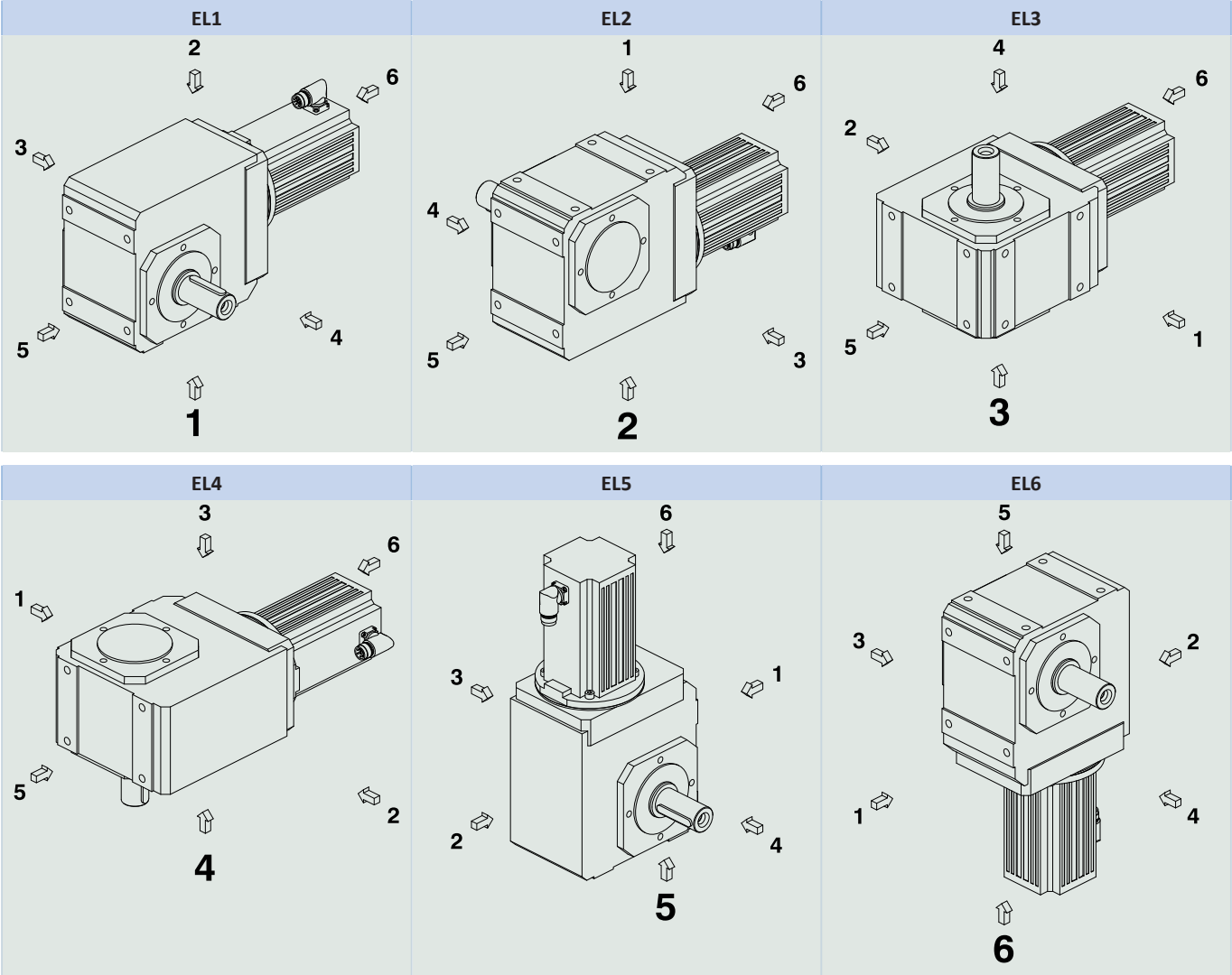
Posiciones de montaje de los reductores de tamaño K1 – K4
