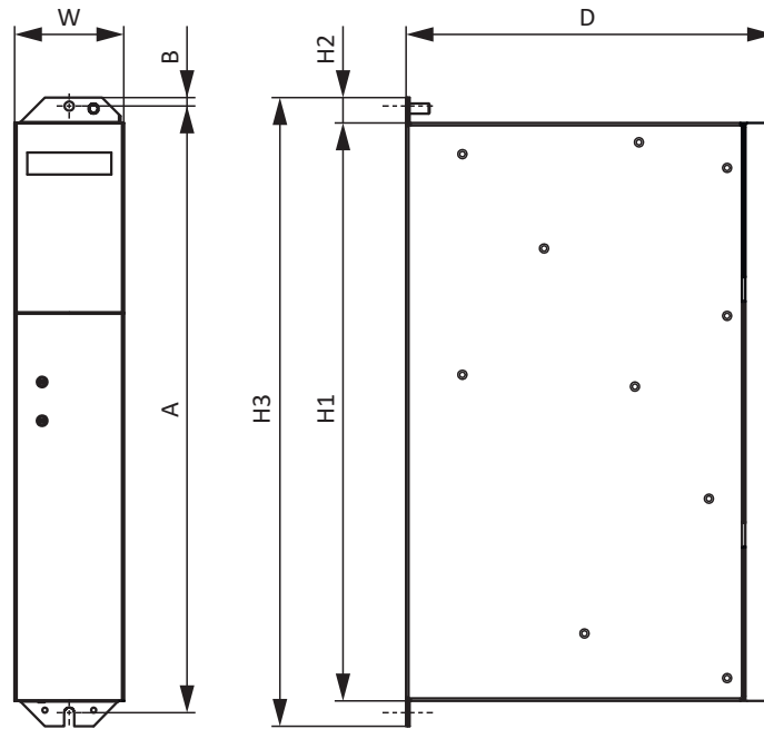
Fig. 1: Esquema de dimensiones PS6A24, PS6A34
