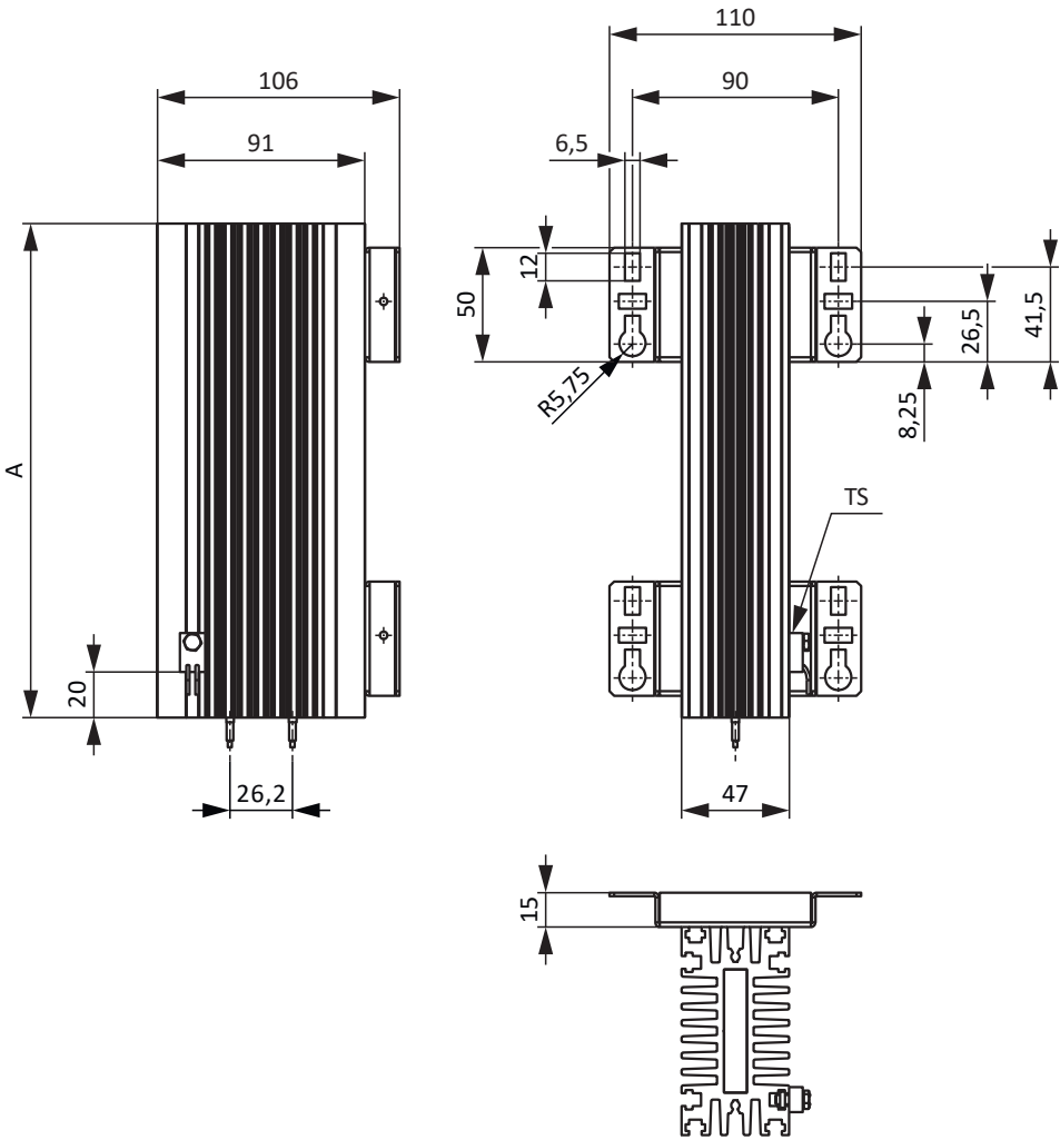
Fig. 10: Esquema de dimensiones KWADQU con MWS310L
