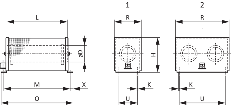
Fig. 4: Esquema de dimensiones FZMU (1), FZZMU (2)
