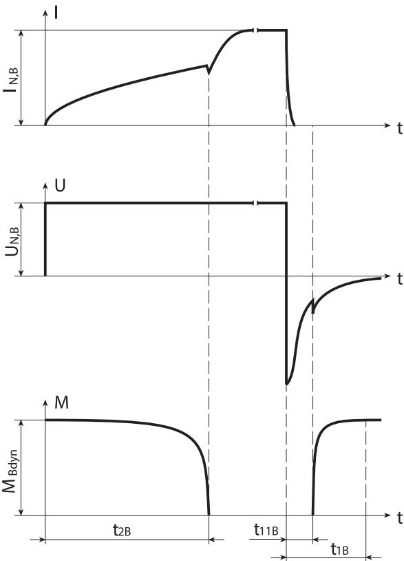
Fig. 3: Comportamiento de conmutación del freno de retención
