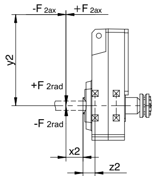
Fig. 2: Puntos de incisión de la fuerza para el eje hueco
