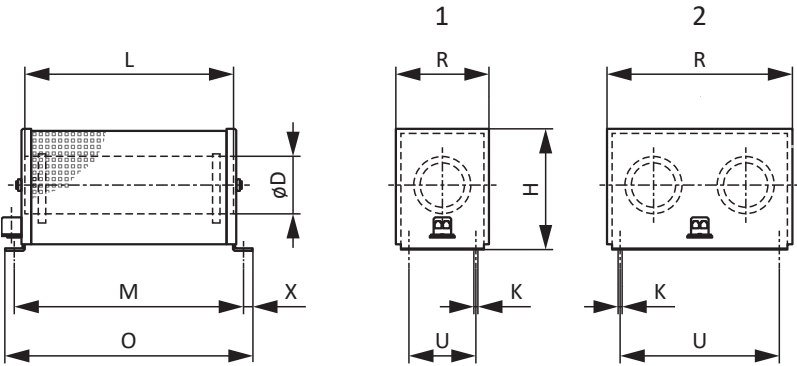
Fig. 3: Esquema de dimensiones FZMU (1), FZZMU (2)
