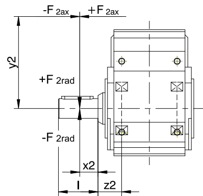
Fig. 1: Puntos de incisión de la fuerza para el eje macizo
