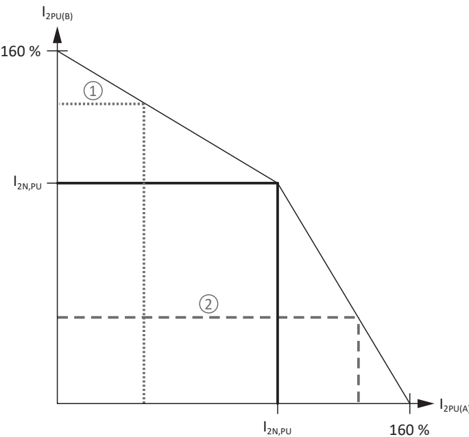
Fig. 3: Carga con terminación simple en reguladores de dos ejes
