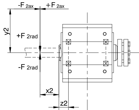
Fig. 2: Puntos de incisión de la fuerza para el eje hueco
