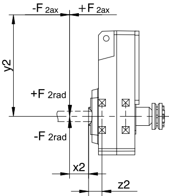
圖 4: 空心軸受力點
