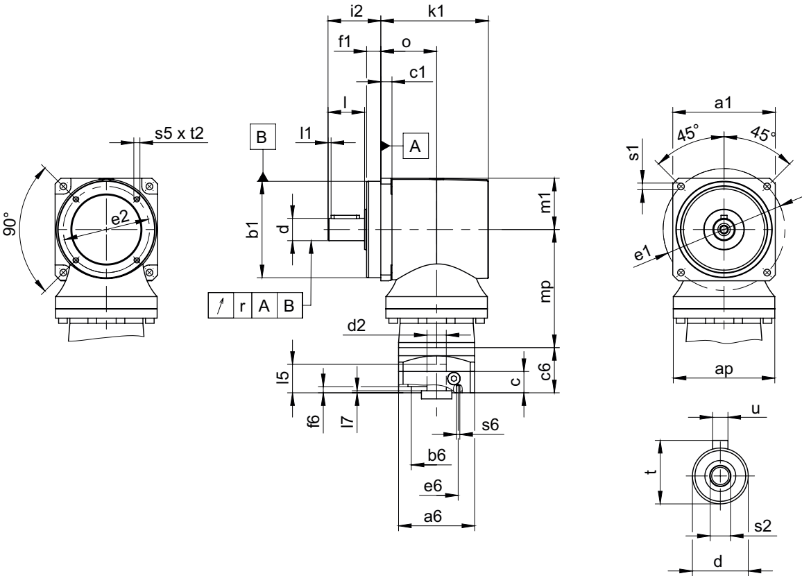
減速機尺寸
