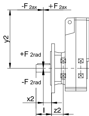
圖 3: 實心軸受力點
