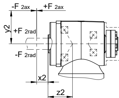
圖 4: 帶有收縮盤的空心軸的受力點
