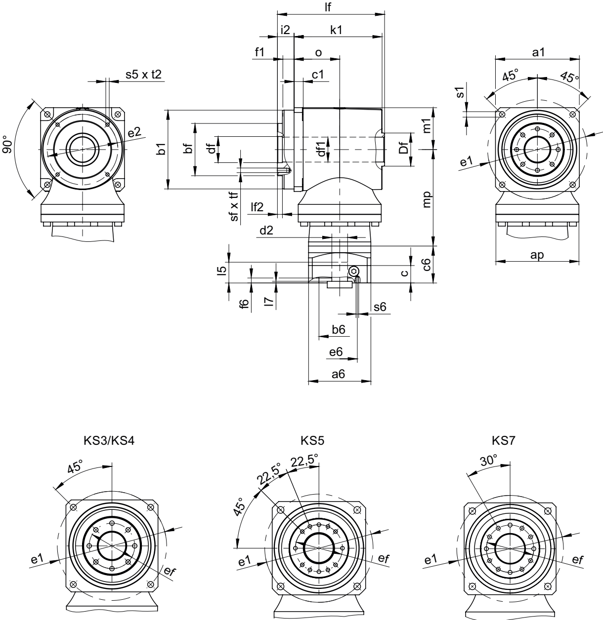
減速機尺寸
