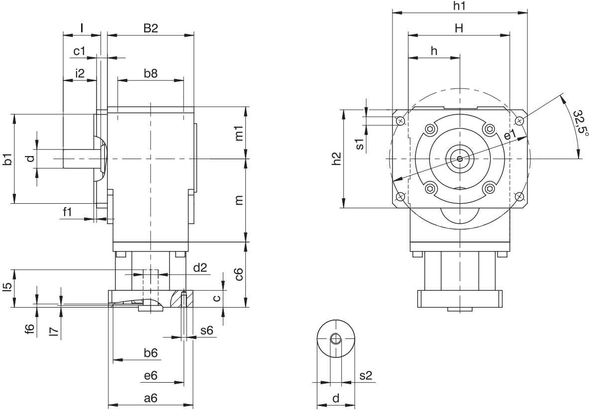
減速機尺寸
