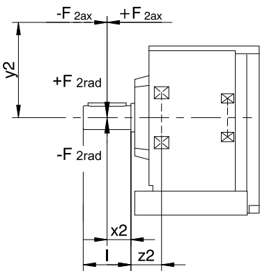
圖 3: 受力點
