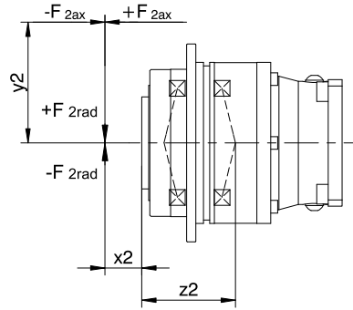
圖 3: 受力點
