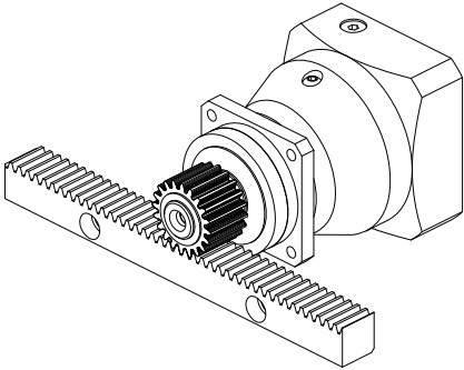
圖 3: 推薦軸承分配 S（例如針對直齒）
