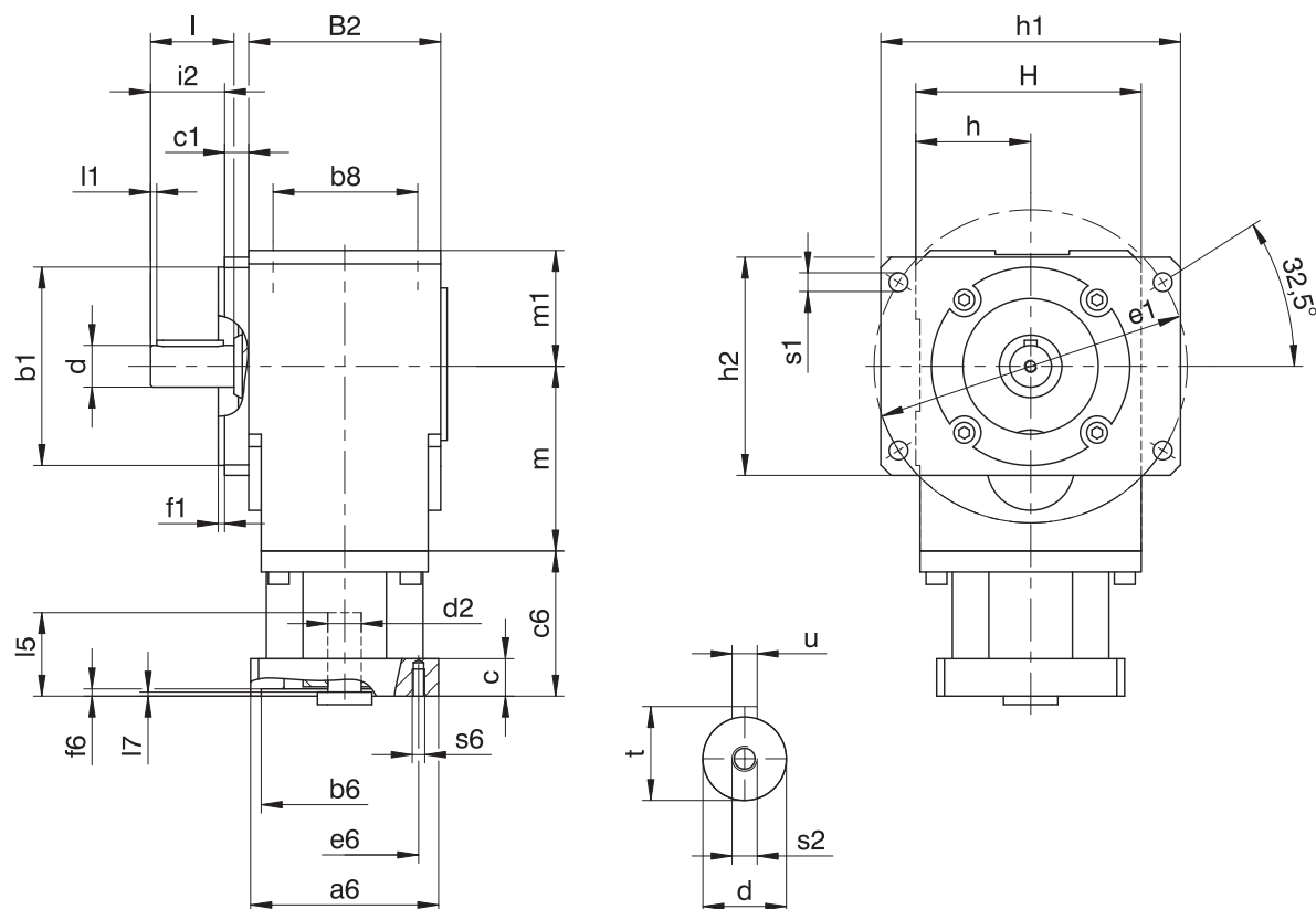
減速機尺寸
