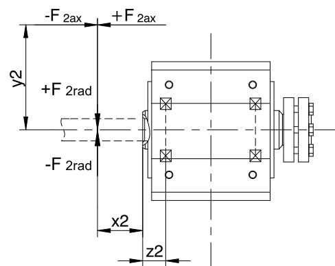
圖 3: 空心軸受力點
