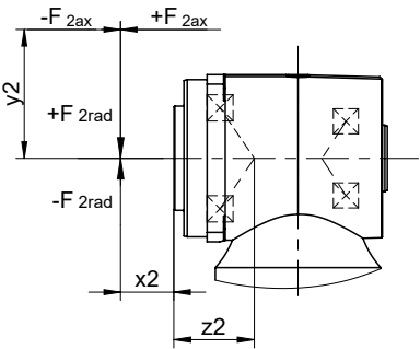
圖 3: 法蘭空心軸受力點
