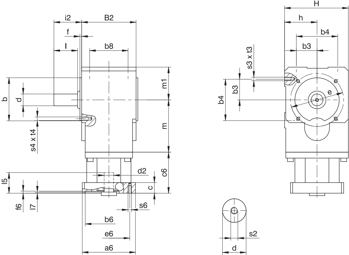
減速機尺寸
