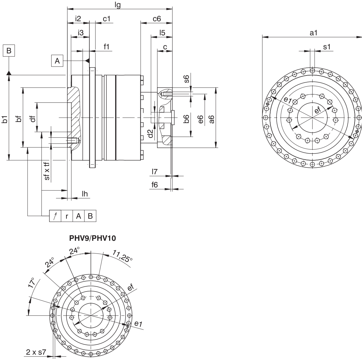
減速機尺寸
