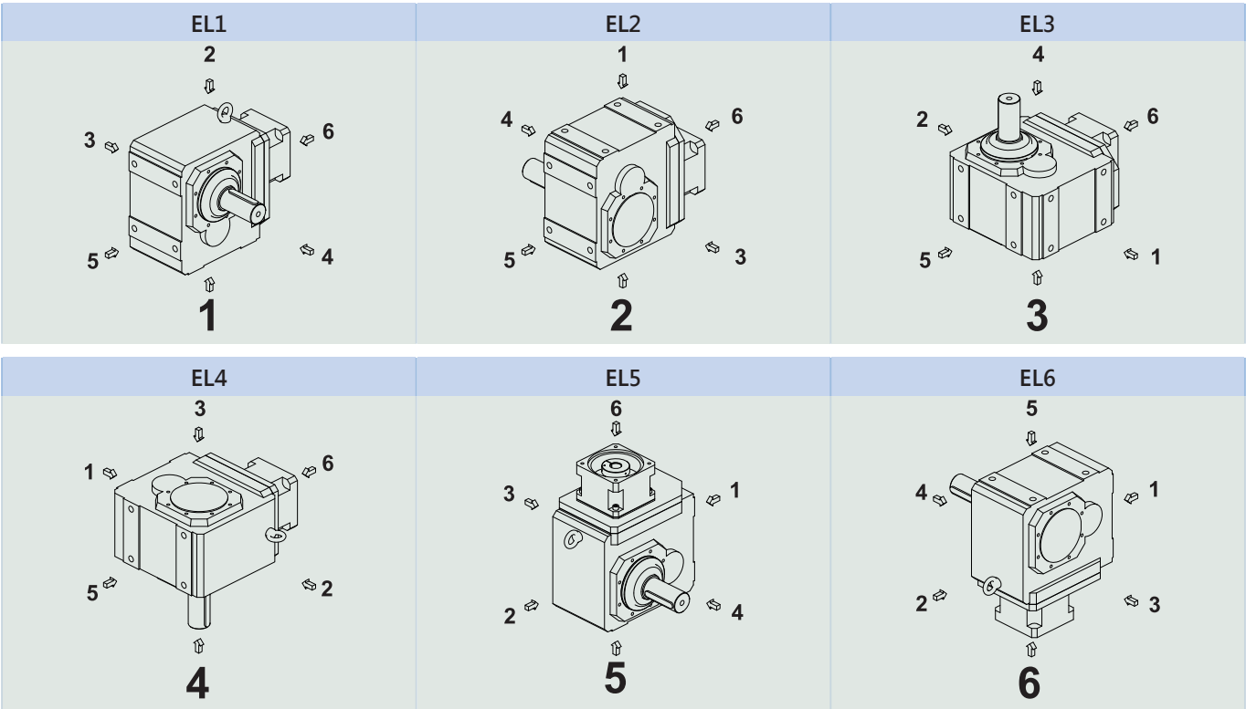
減速器結構尺寸 K5 – K10 安裝方向
