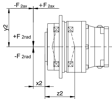
圖 2: 受力點
