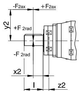
圖 6: 受力點
