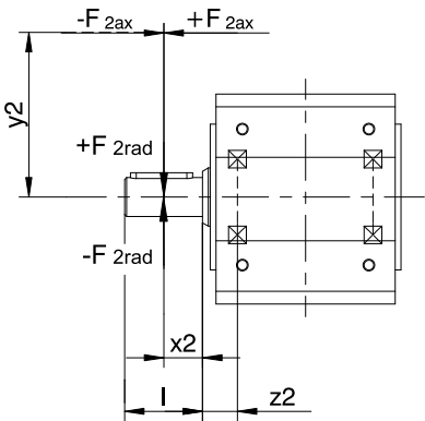
圖 2: 實心軸受力點
