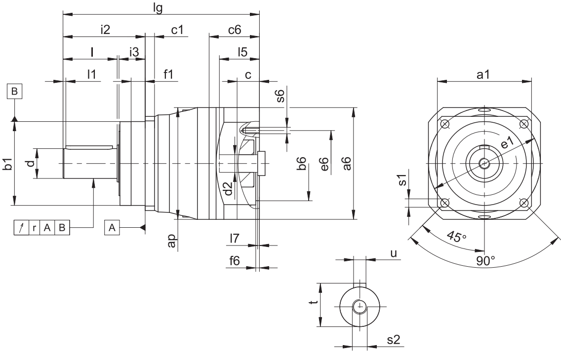
減速機尺寸
