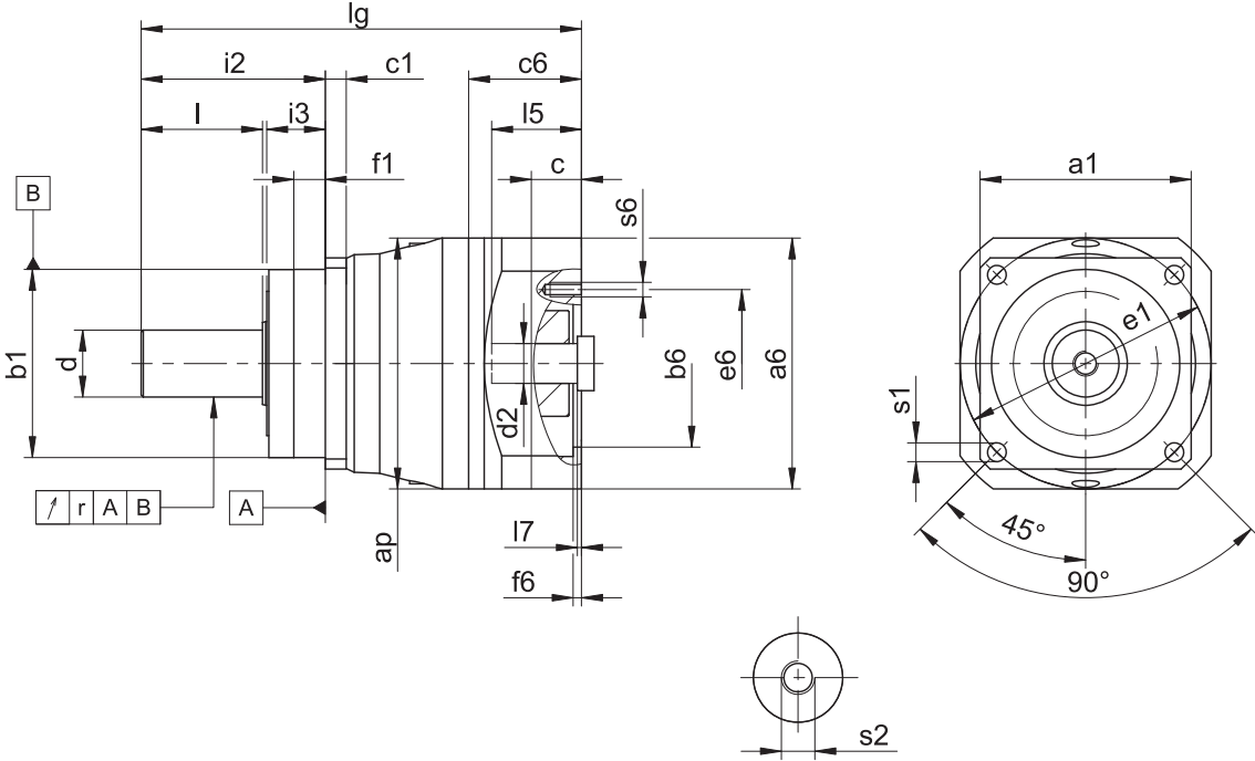
減速機尺寸
