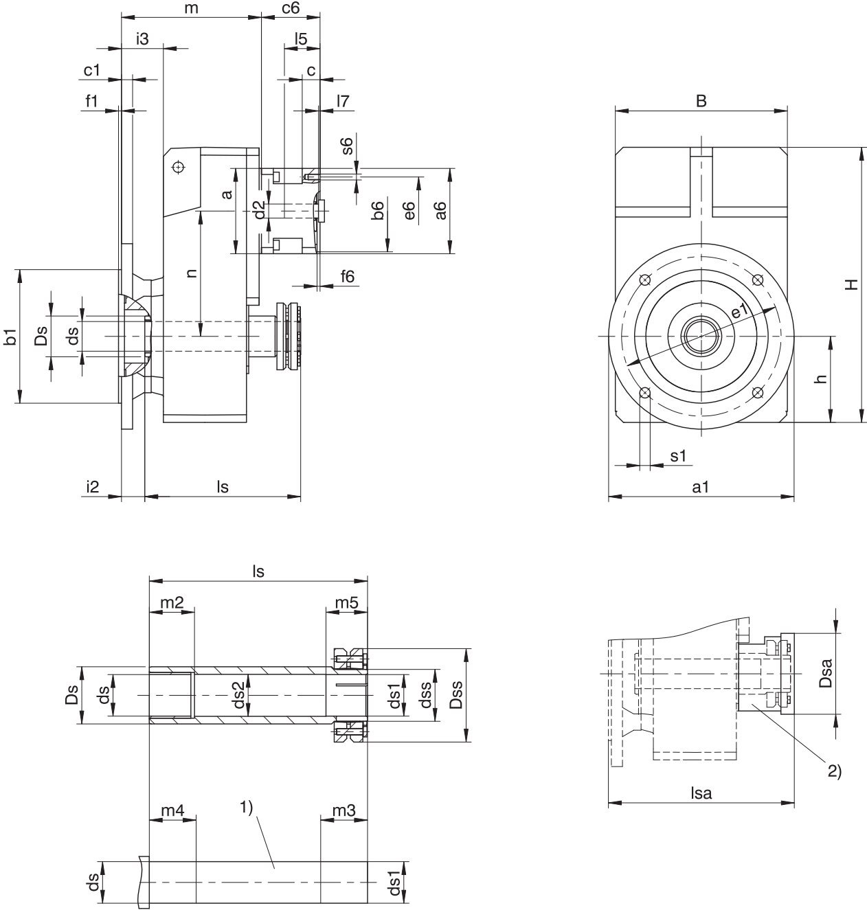
減速機尺寸
