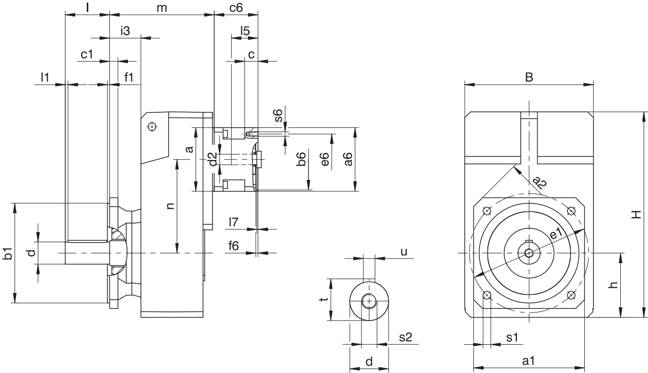
減速機尺寸
