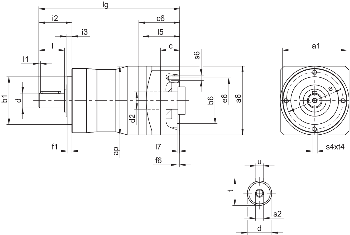
減速機尺寸
