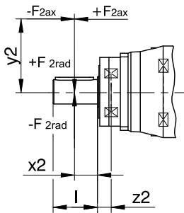
圖 5: 受力點
