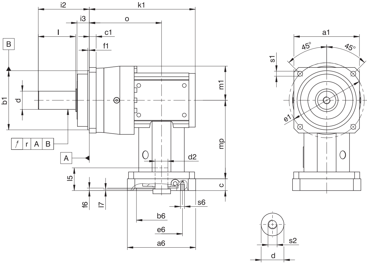
減速機尺寸
