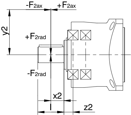
圖 2: 受力點
