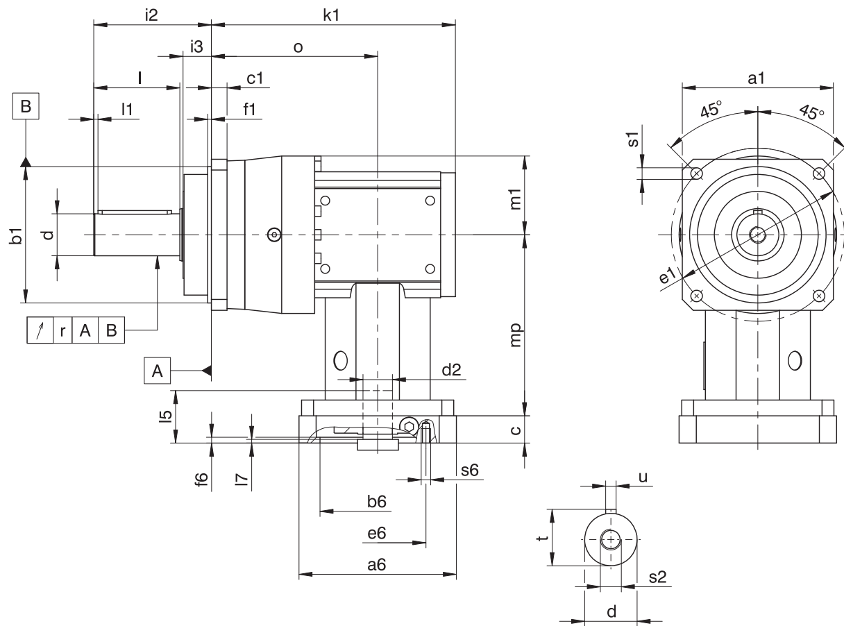
減速機尺寸
