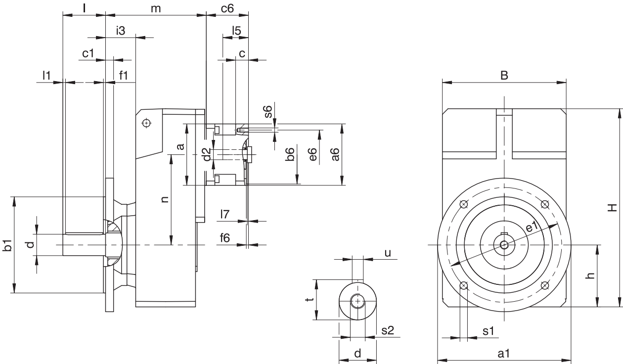
減速機尺寸
