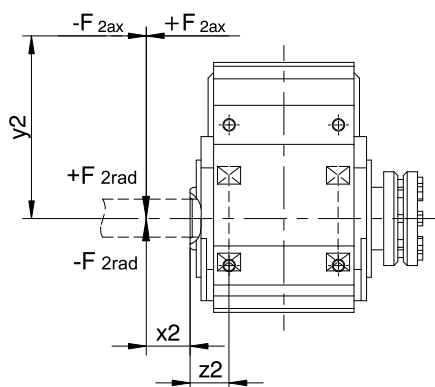
圖 4: 空心軸受力點
