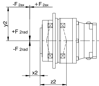
圖 2: 受力點
