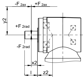
圖 5: 實心軸受力點
