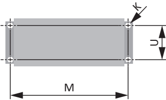
Fig. 22: Plan de perçage FZMU, FZZMU
