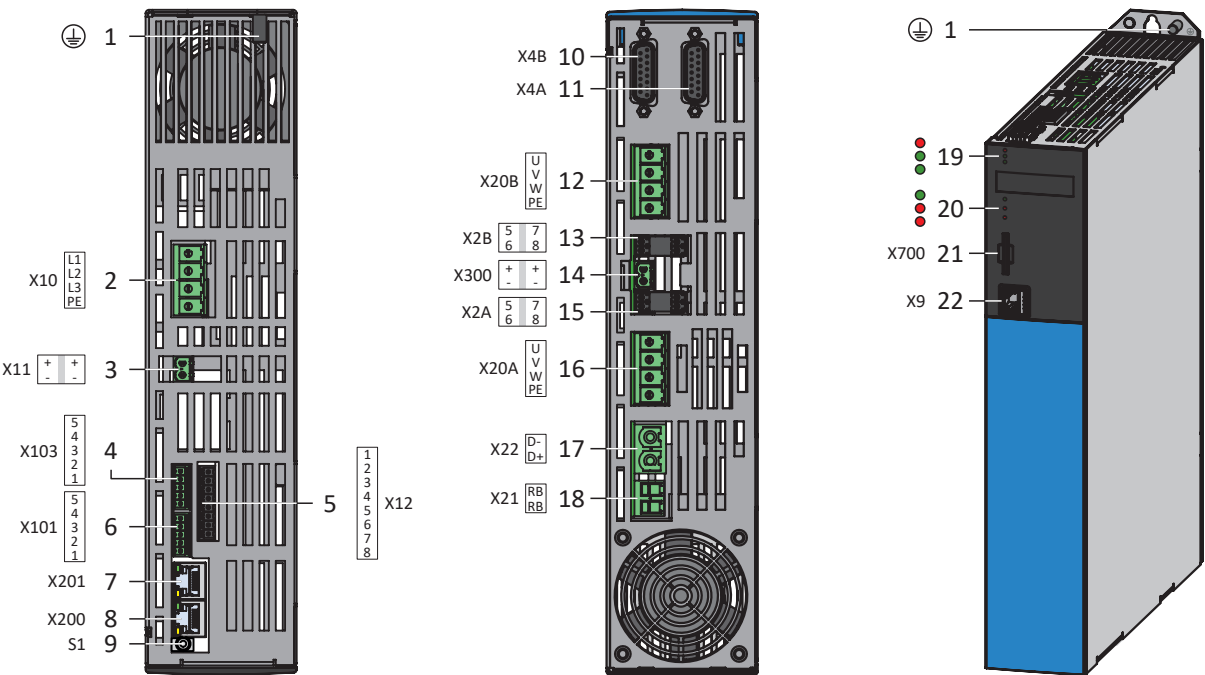
Fig. 28: Schéma de raccordement à l'exemple du SC6A162
