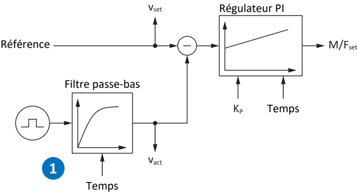
Fig. 37: Régulateur de vitesse – filtre pour la vitesse réelle
