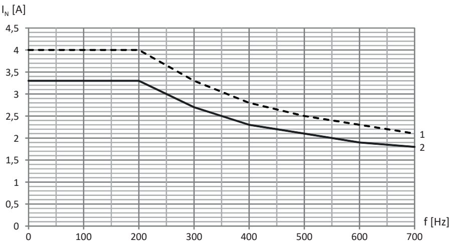
Fig. 12: R duction du courant nominal en fonction de la cadence, TEP3720-0ES41
