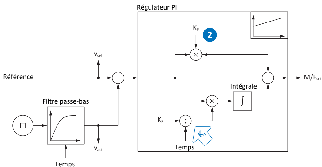
Fig. 38: Régulateur de vitesse – coefficient d'action proportionnelle
