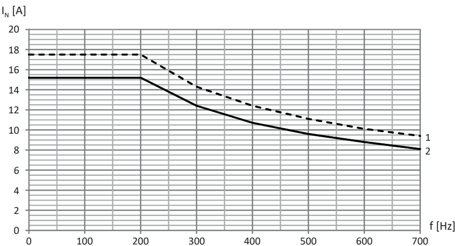
Fig. 13: R duction du courant nominal en fonction de la cadence, TEP3820-0CS41
