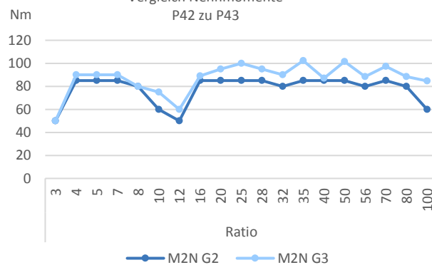
Vergleich Nennmomente P42 zu P43
