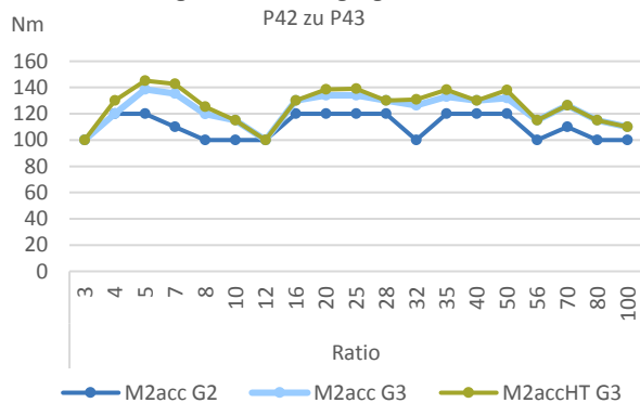
Vergleich Beschleunigungsmomente P42 zu P43
