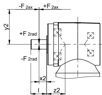
図 5: ソリッドシャフト用の荷重の作用点
