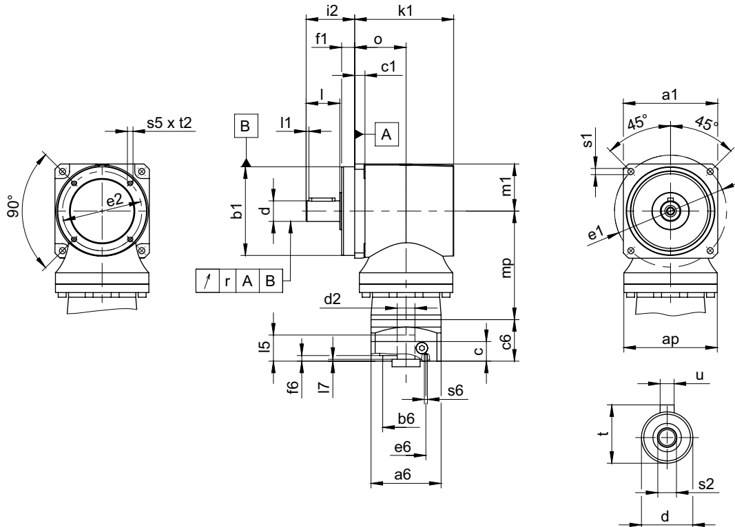
減速機の寸法
