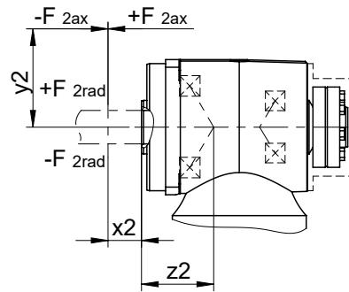
図 4: シュリンクディスク付き中空シャフト用の荷重の作用点
