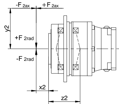
図 3: 荷重の作用点
