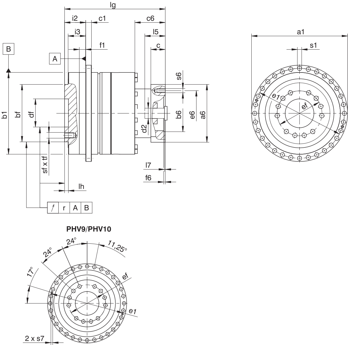
減速機の寸法
