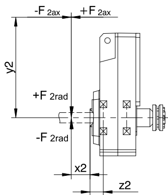
図 4: 中空シャフト用の荷重の作用点
