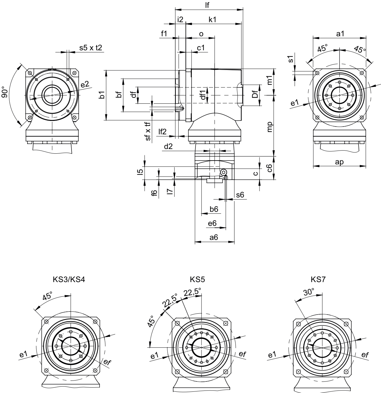
減速機の寸法
