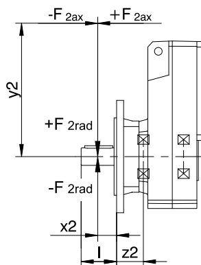
図 3: ソリッドシャフト用の荷重の作用点
