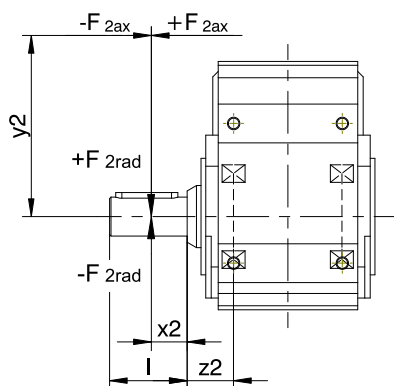
図 3: ソリッドシャフト用の荷重の作用点
