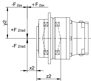
図 2: 荷重の作用点
