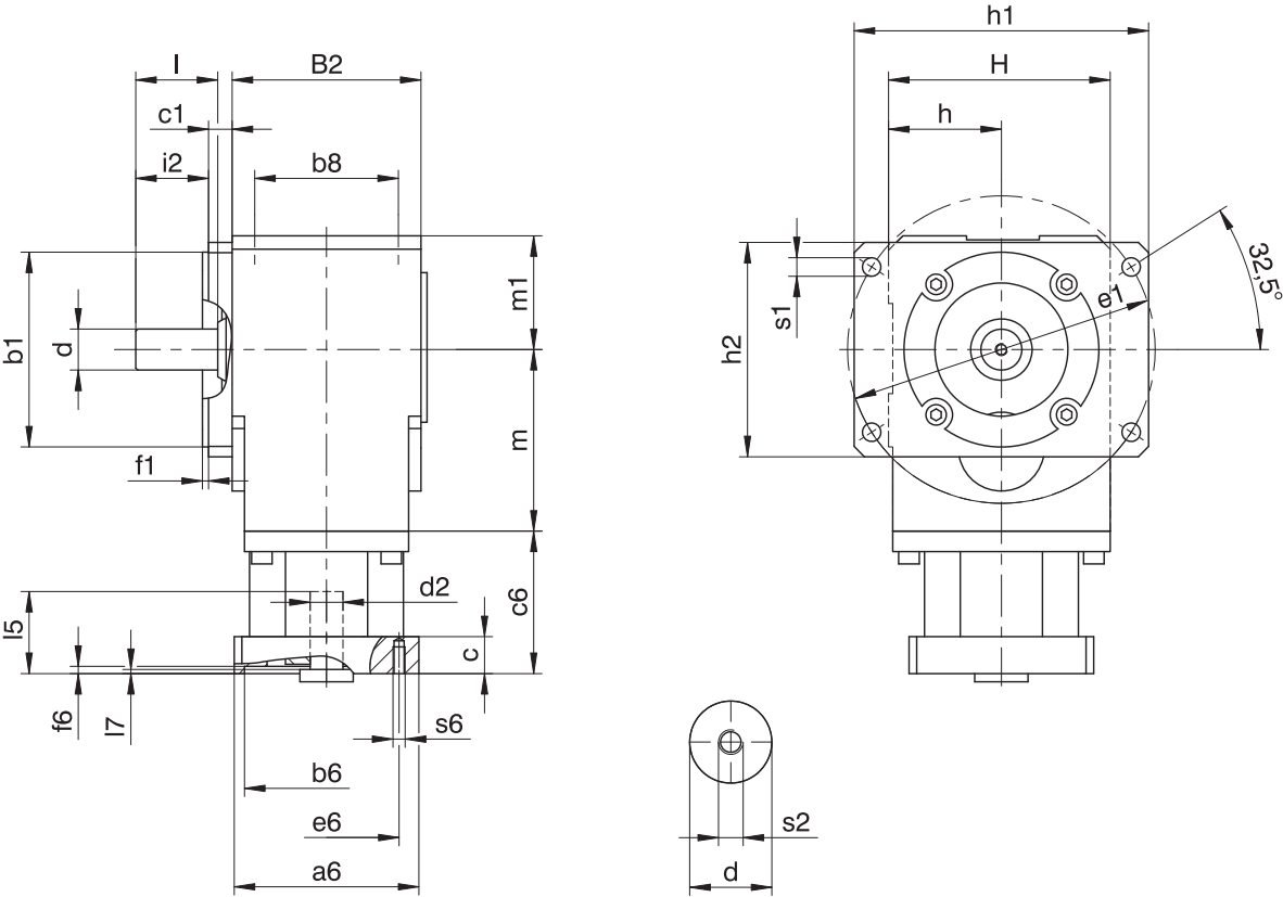
減速機の寸法
