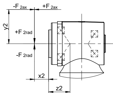
図 3: フランジ中空シャフト用の荷重の作用点
