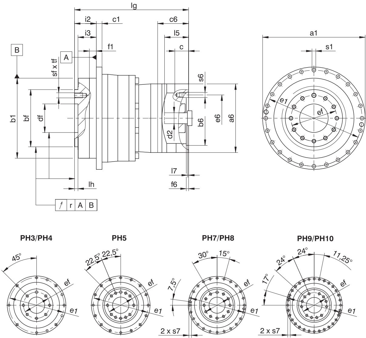
減速機の寸法
