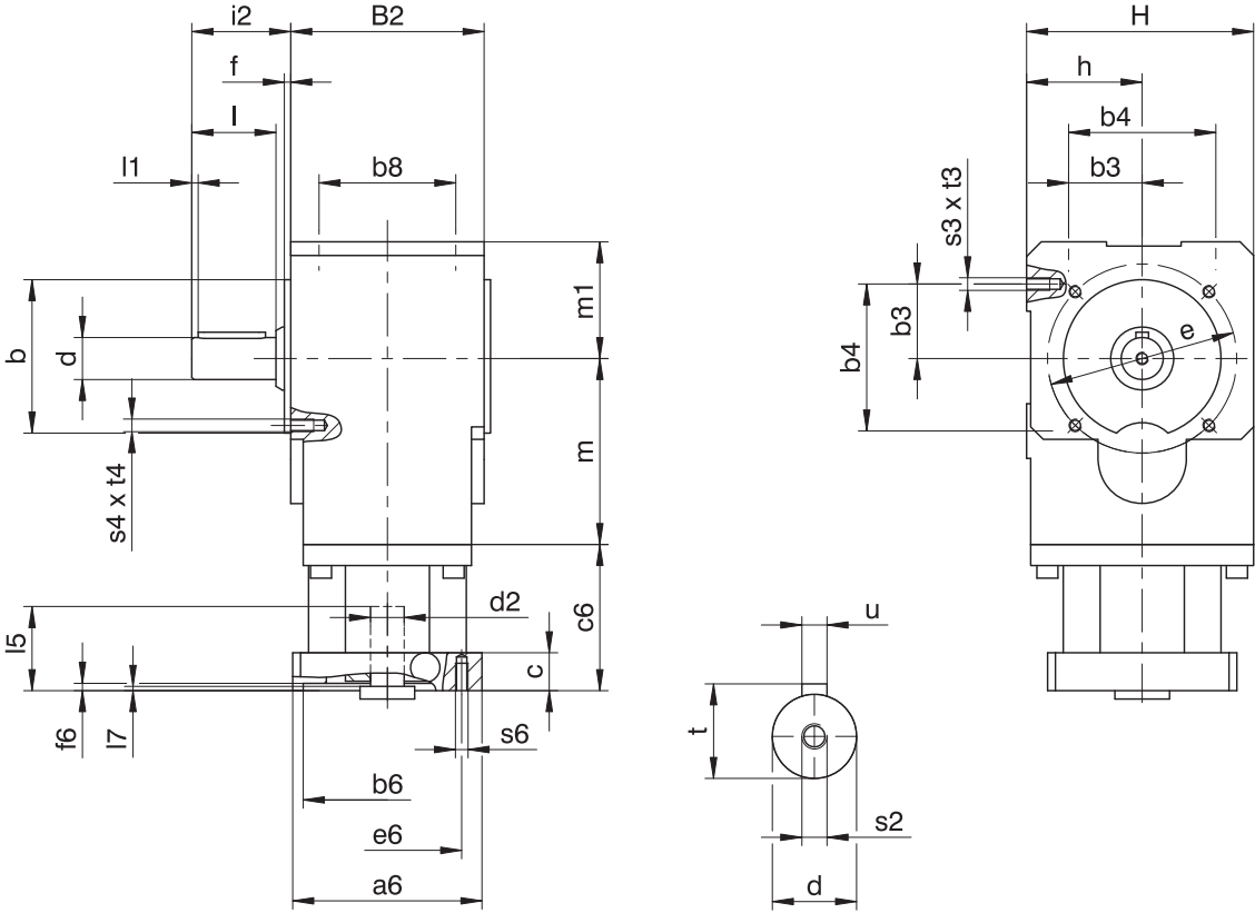
減速機の寸法
