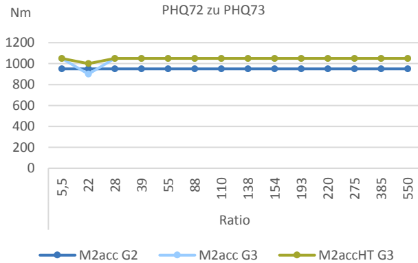
Vergleich Beschleunigungsmomente PHQ72 zu PHQ73
