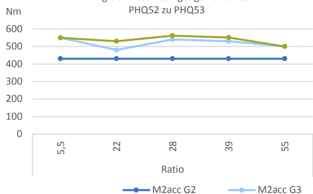
Vergleich Beschleunigungsmomente PHQ52 zu PHQ53
