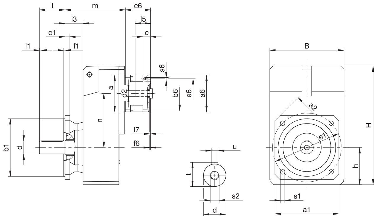
Dimensioni riduttori
