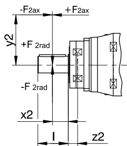
Fig. 6: Punti di applicazione della forza
