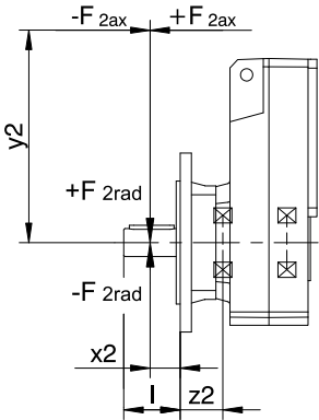
Fig. 3: Punti di applicazione della forza per l'albero pieno
