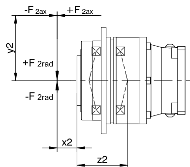
Fig. 2: Punti di applicazione della forza
