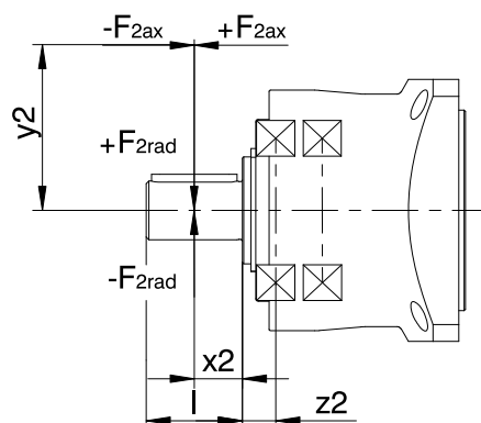
Fig. 2: Punti di applicazione della forza
