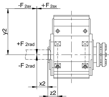
Fig. 4: Punti di applicazione della forza per l'albero cavo
