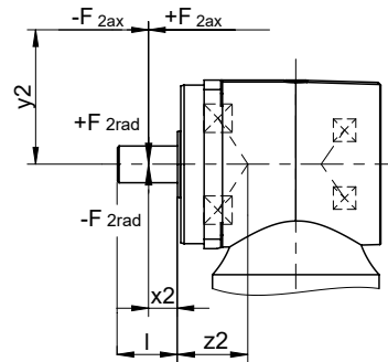
Fig. 5: Punti di applicazione della forza per l'albero pieno
