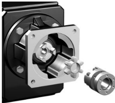
Fig. 2: Accoppiamento ad innesto senza gioco
