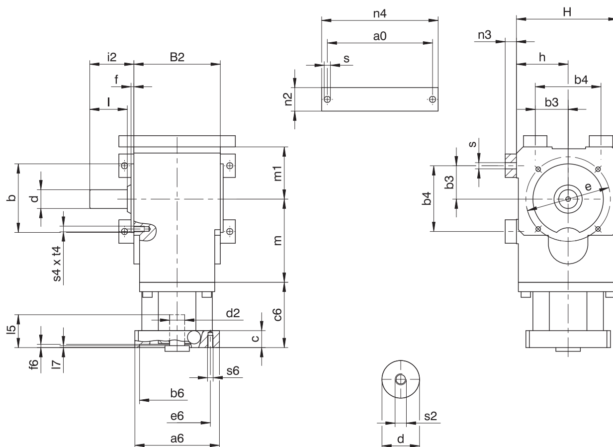
Dimensioni riduttori
