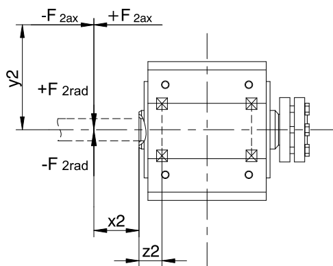
Fig. 3: Punti di applicazione della forza per l'albero cavo
