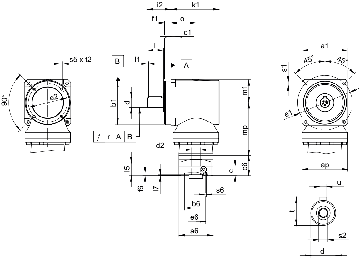
Dimensioni riduttori
