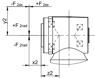
Fig. 3: Punti di applicazione della forza per l'albero cavo flangiato
