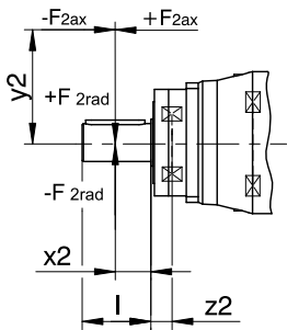
Fig. 6: Punti di applicazione della forza
