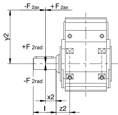
Fig. 3: Punti di applicazione della forza per l'albero pieno
