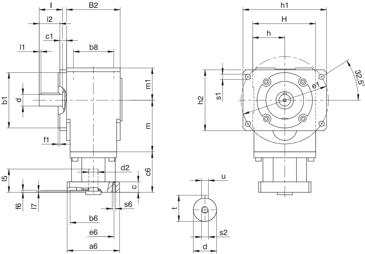
Dimensioni riduttori
