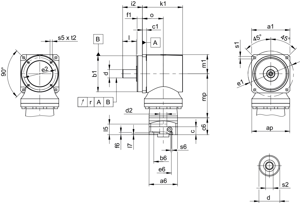
Dimensioni riduttori
