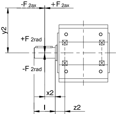
Fig. 2: Punti di applicazione della forza per l'albero pieno
