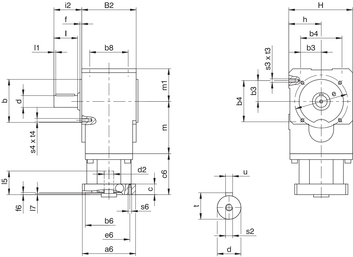
Dimensioni riduttori
