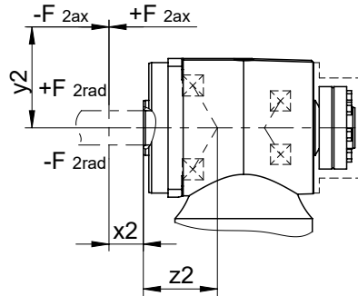
Fig. 4: Punti di applicazione della forza per l'albero cavo con anello calettatore
