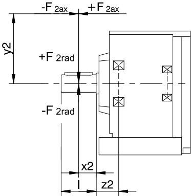
Fig. 3: Punti di applicazione della forza
