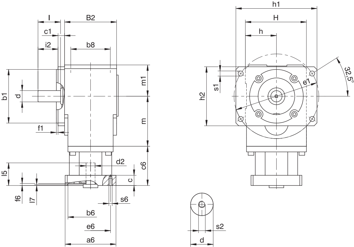
Dimensioni riduttori
