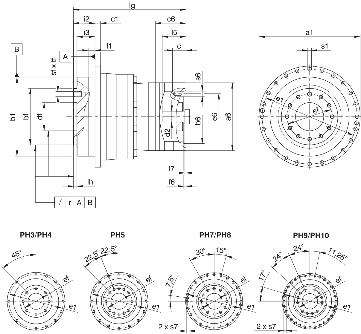
Dimensioni riduttori
