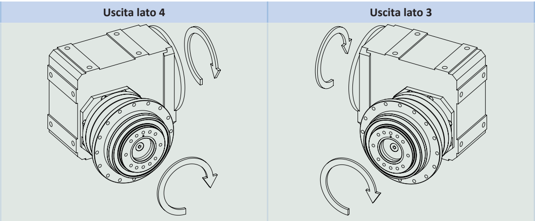
Le figure mostrano la posizione di montaggio EL1.
