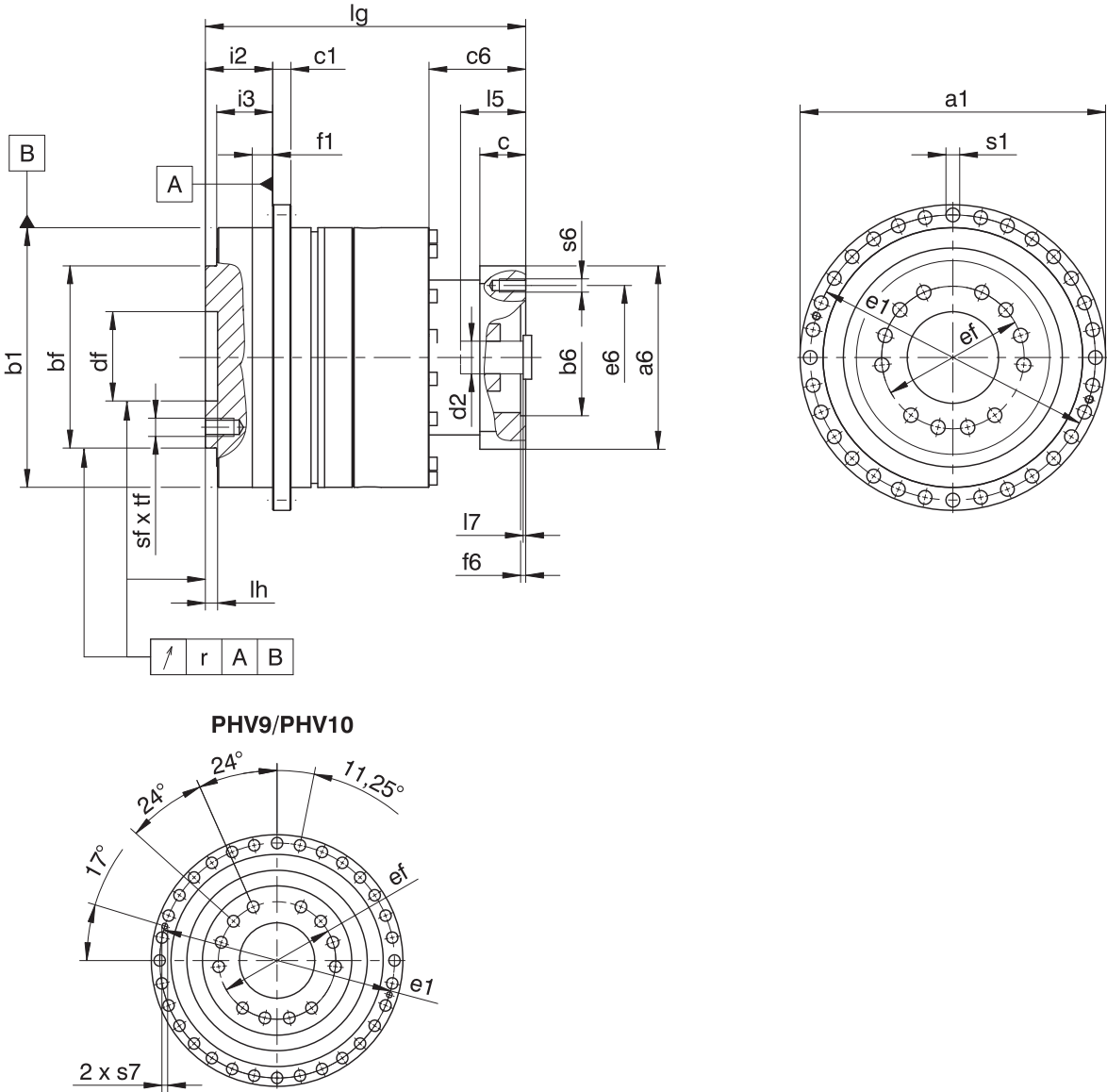
Dimensioni riduttori
