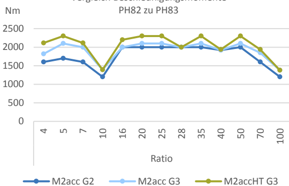
Vergleich Beschleunigungsmomente PH82 zu PH83
