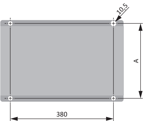
Abb. 30: Bohrplan FGFKU
