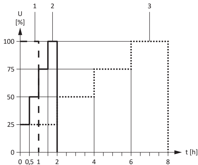
Abb. 25: Spannungshöhen in Abhängigkeit von der Lagerungszeit
