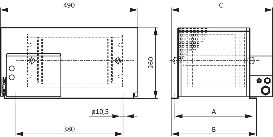
Abb. 10: Maßzeichnung FGFKU
