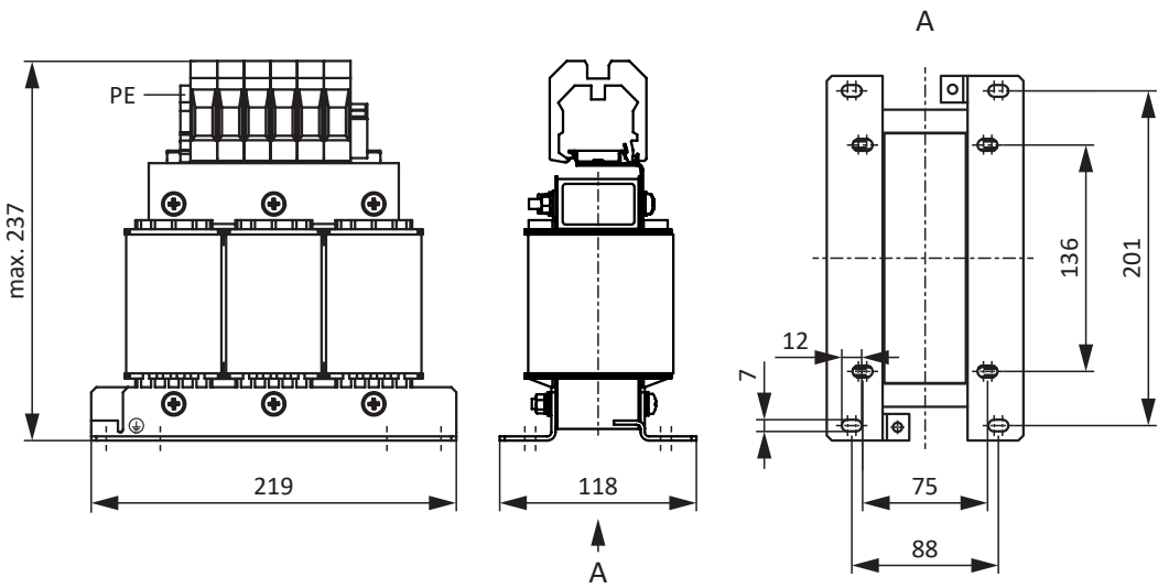
Abb. 11: Maßzeichnung Netzdroessel
