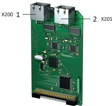
Abb. 50: Anschlussübersicht Kommunikationsmodul PN6
