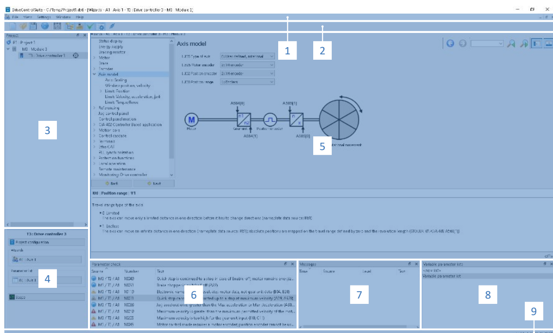
Abb. 69: DS6: Programmoberfläche
