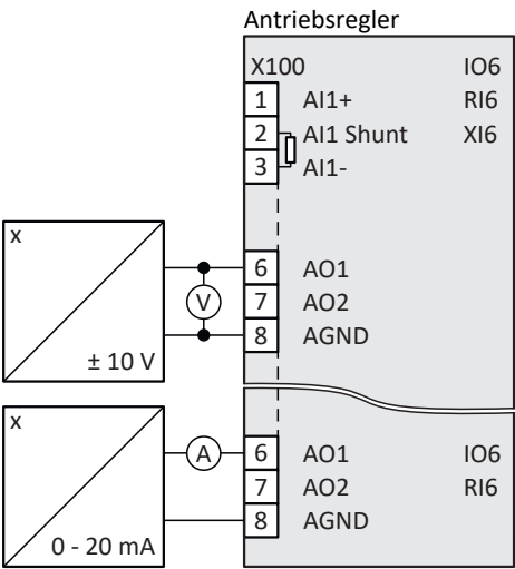
Abb. 55: X100: Anschlussbeispiel Aktuator
