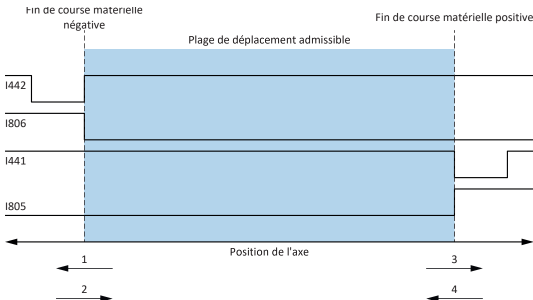
Fig. 22: Fins de course matérielles : mémoire des fins de course
