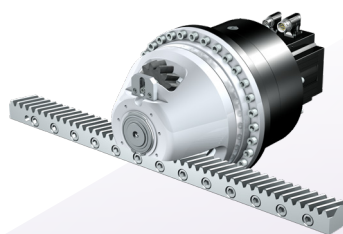
带同步伺服电机的齿轮齿条传动 ZTRSPH、ZTRSPHQ、ZTRSPHV 模数：3 - 8 mm 进给力：5 - 124 kN 进给速度：0.11 - 3.6 m/s 大进给力，确保最大功率密度。
