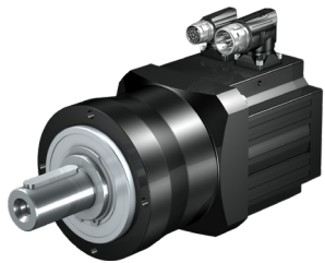
行星齿轮减速电机 PE 加速力矩：17 - 250 Nm 齿隙：8 - 13 弧分 经济的斜齿款。
