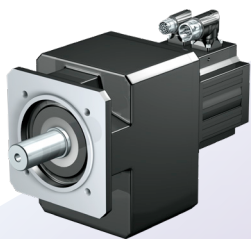
斜齿轮减速电机 C 加速力矩：47 - 8000 Nm 齿隙：10 - 20 弧分 外形美观。动态。 经典的斜齿款。
