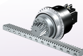
带同步伺服电机的齿轮齿条传动 ZTRPH、 ZTRPHV 模数：2 - 6 mm 进给力：1.9 - 67 kN 进给速度：0.11 - 4.3 m/s 高性能，适用于要求严苛的驱动方案。
