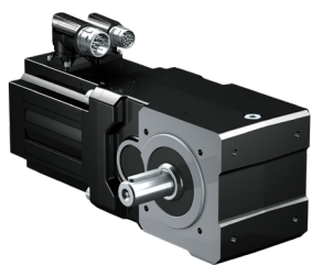
螺旋伞齿轮减速电机 KL 加速力矩：22 - 65 Nm 齿隙：16 - 25 弧分 完全无轴偏移。
