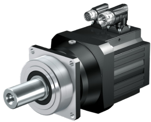
行星齿轮减速电机 P 加速力矩：21 - 3450 Nm 齿隙：1 - 8 弧分 精度高，运行平稳性出色。
