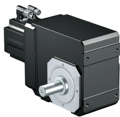
螺旋伞齿轮减速电机 K 加速力矩：60 - 13200 Nm 齿隙：1,5 - 12 弧分 间隙稳定性尤为出色。
