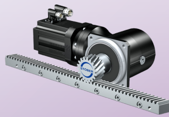
带同步伺服电机的齿轮齿条传动 ZVKS 模数：2 - 4 mm 进给力：1.3 - 11 kN 进给速度：0.08 - 3 m/s 高度灵活 用于自动化系统和机械手装置。
