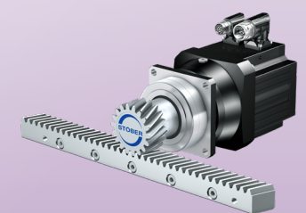
带同步伺服电机的齿轮齿条传动 ZVP 模数：2 - 4 mm 进给力：0.8 - 11 kN 进给速度：0.1 - 5.3 m/s 精确度高，适合各种典型的伺服应用。
