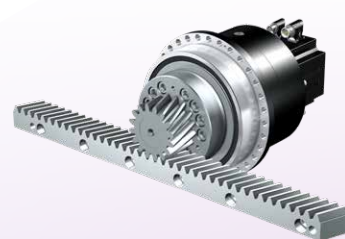
Azionamenti a cremagliera con servomotori sincroni ZTRPH, ZTRPHV Modulo: 2–6 mm Forza di avanzamento: 1,9–67 kN Velocità di avanzamento: 0,11–4 m/s Prestazioni elevate per sistemi di trasmissione esigenti.
