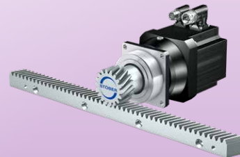
Azionamento a cremagliera con servomotore sincrono ZVP Modulo: 2–4 mm Forza di avanzamento: 0,8–11 kN Velocità di avanzamento: 0,1–4,5 m/s Alta precisione per le tipiche applicazioni servoassistite.
