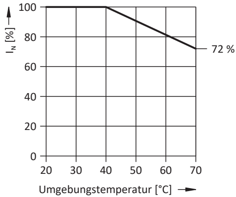
Abb. 22: Derating des Nennstroms in Abhängigkeit von der Umgebungstemperatur
