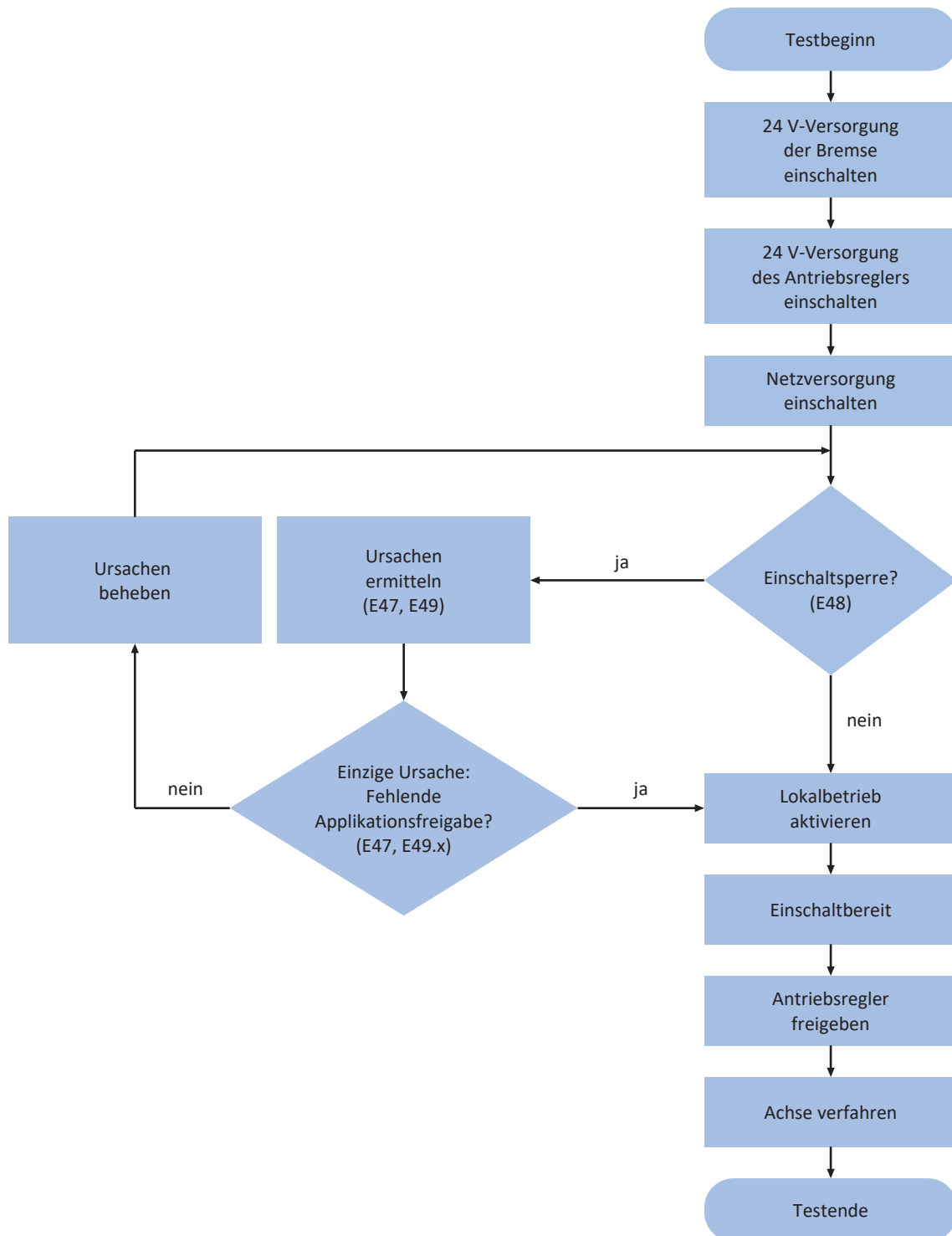
Abb. 58: Schematischer Testablauf Verdrahtungs- und Funktionstest
