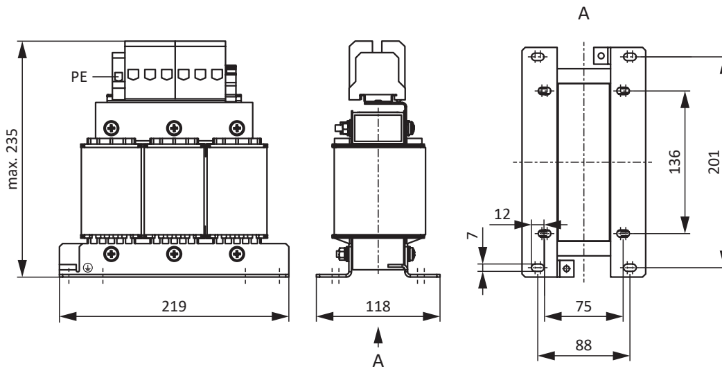
Abb. 11: Maßzeichnung Netzdrössel
