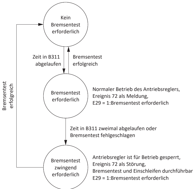
Abb. 78: Zustandsmaschine des Bremsenmanagements
