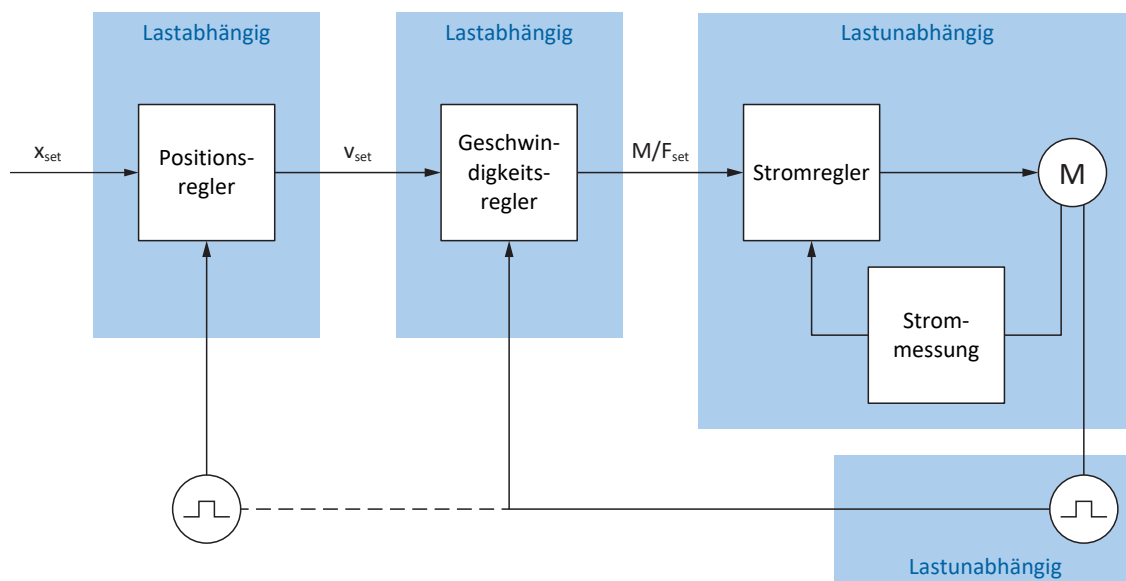
Abb. 59: Aufbau der Regelungskaskade
