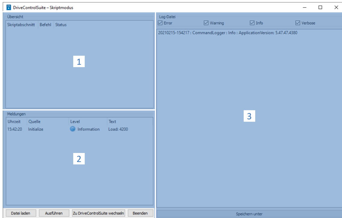
Abb. 100: Skriptmodus: Programmoberfläche
