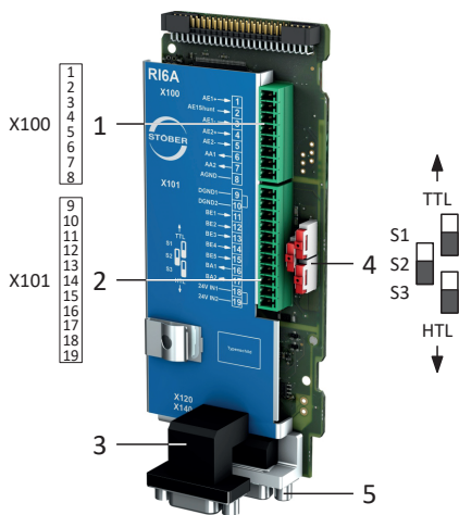
Abb. 52: Anschlussübersicht Klemmenmodul RI6
