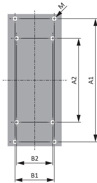
Abb. 32: Bohrplan TEP
