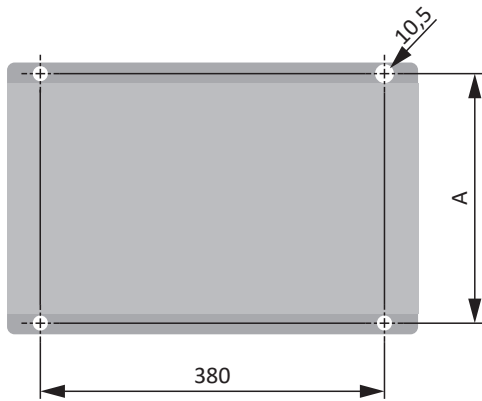
Abb. 30: Bohrplan FGFKU
