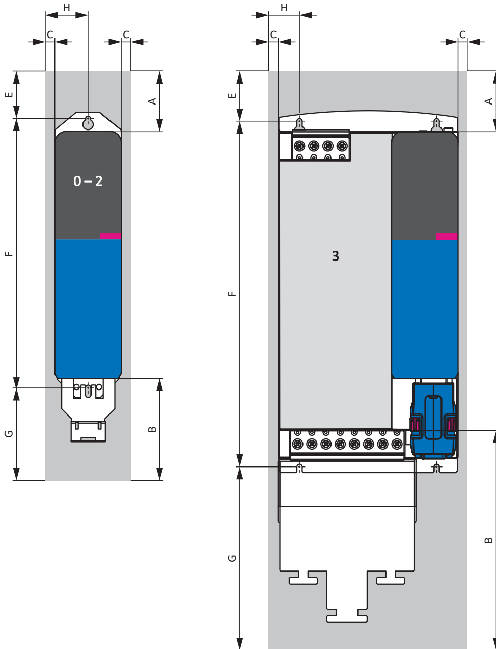
Abb. 26: Mindestfreiräume
