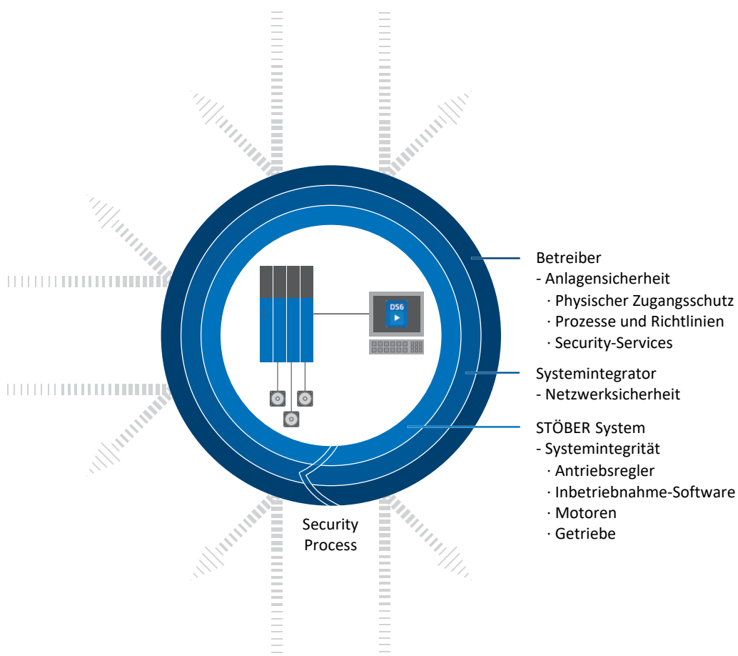
Abb. 1: Defense-in-Depth-Konzept
